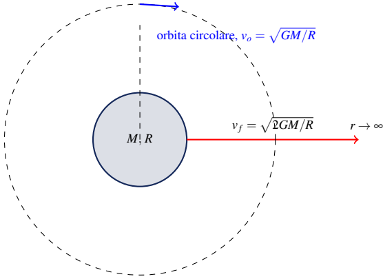
Figure 4: Schema concettuale: traiettoria radiale di fuga (freccia rossa) rispetto alla traiettoria orbitale circolare a raggio R (freccia blu tangente, cerchio tratteggiato), con v_f = \sqrt{2}v_o .
