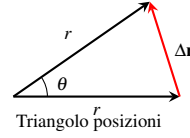
Triangolo \mathbf{r} posizioni
