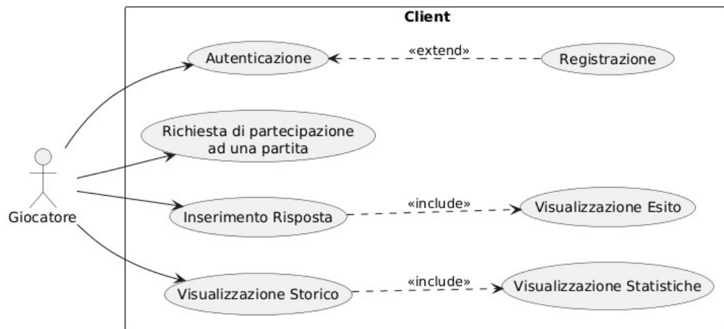
Diagramma dei casi d'uso per il client
