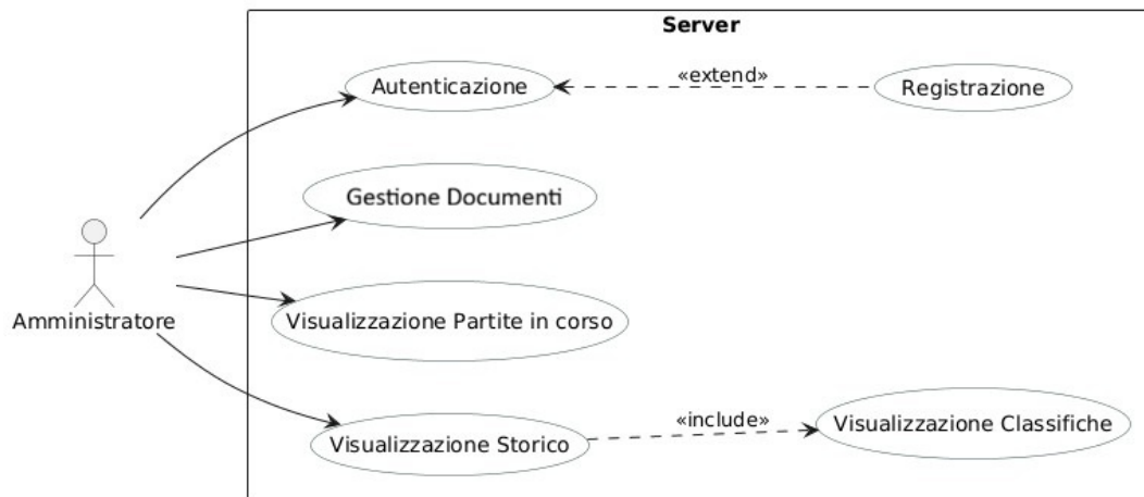
Diagramma dei casi d'uso per il server
