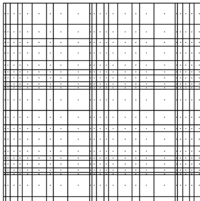
Figura 2.8: Zoom da malha m-tree.
