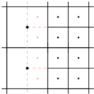
Figura 2.6: Malha 2D com células fantasmas.
