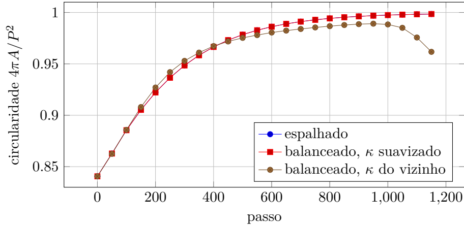
Figura 2: Relaxação da gota elíptica ( Re = 1 , superamortecido). A tensão superficial leva a elipse ao círculo de mesma área de forma monotônica, sem oscilar. É neste caso que a cirurgia dispara pela primeira vez com o solver no circuito, removendo marcadores conforme a frente encurta.
