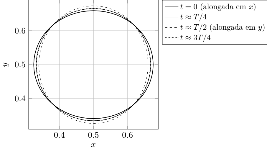
Figura 3: Fases de um período da oscilação do modo n = 2 ( Re = 200 ). A gota troca de eixo maior a cada meio período — é essa troca de sinal que a deformação D = (a - b)/(a + b) registra, e que a circularidade, sempre \leq 1 , não registraria. A amplitude está exagerada pelo recorte dos eixos: a deformação inicial é de 5 %.
