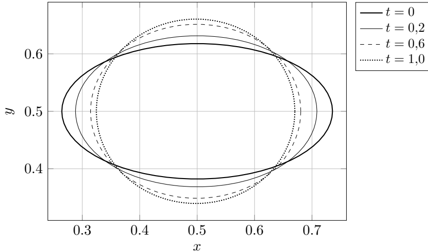
Figura 2: Relaxação da gota elíptica ( Re = 1 , superamortecido). A tensão superficial leva a elipse ao círculo de mesma área de forma monotônica, sem oscilar. É neste caso que a cirurgia dispara pela primeira vez com o solver no circuito, removendo marcadores conforme a frente encurta.
