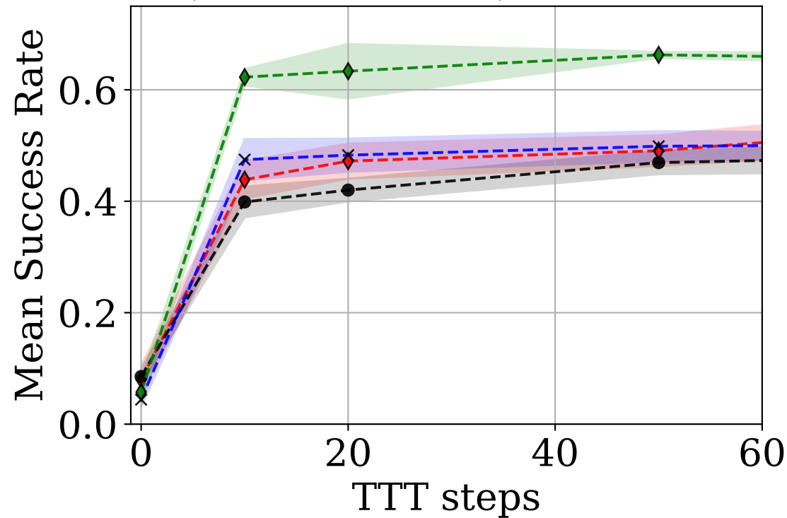
(Humanoidmaze) DDPG-BC
