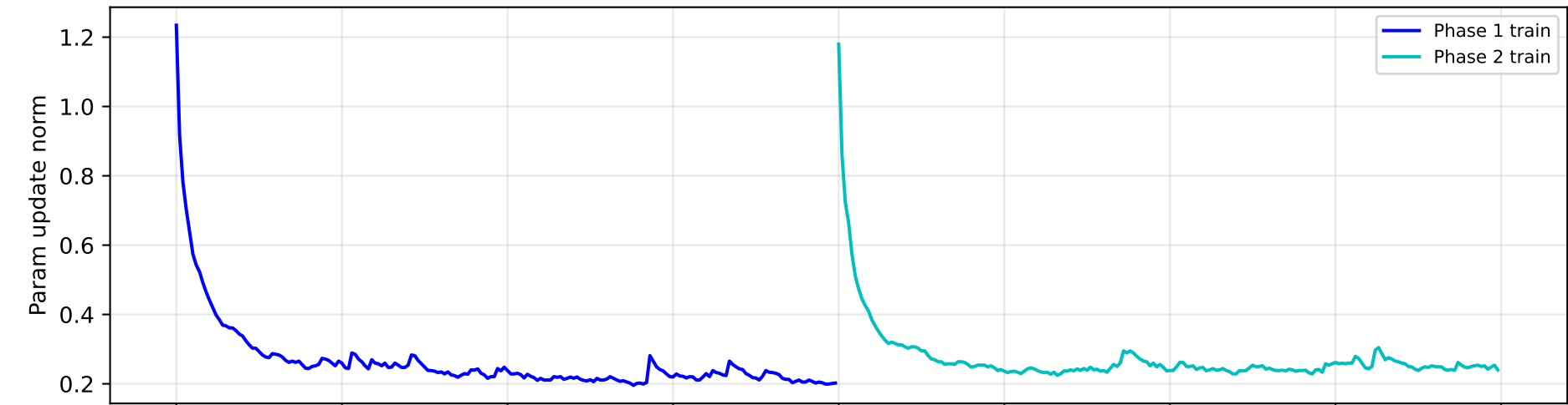
Parameter shift magnitude (L2 norm of updates)
