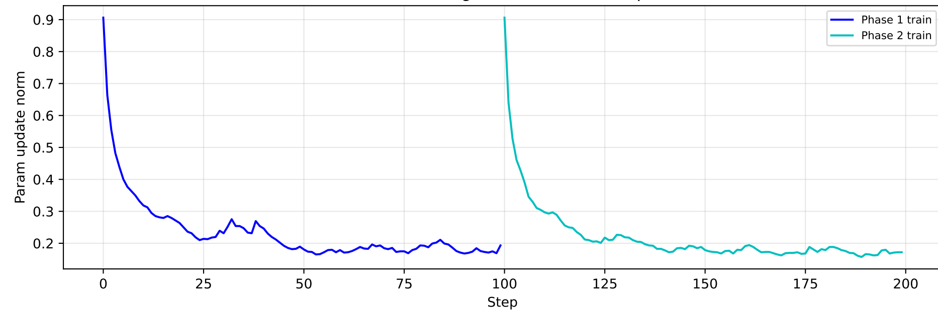
Parameter shift magnitude (L2 norm of updates)
