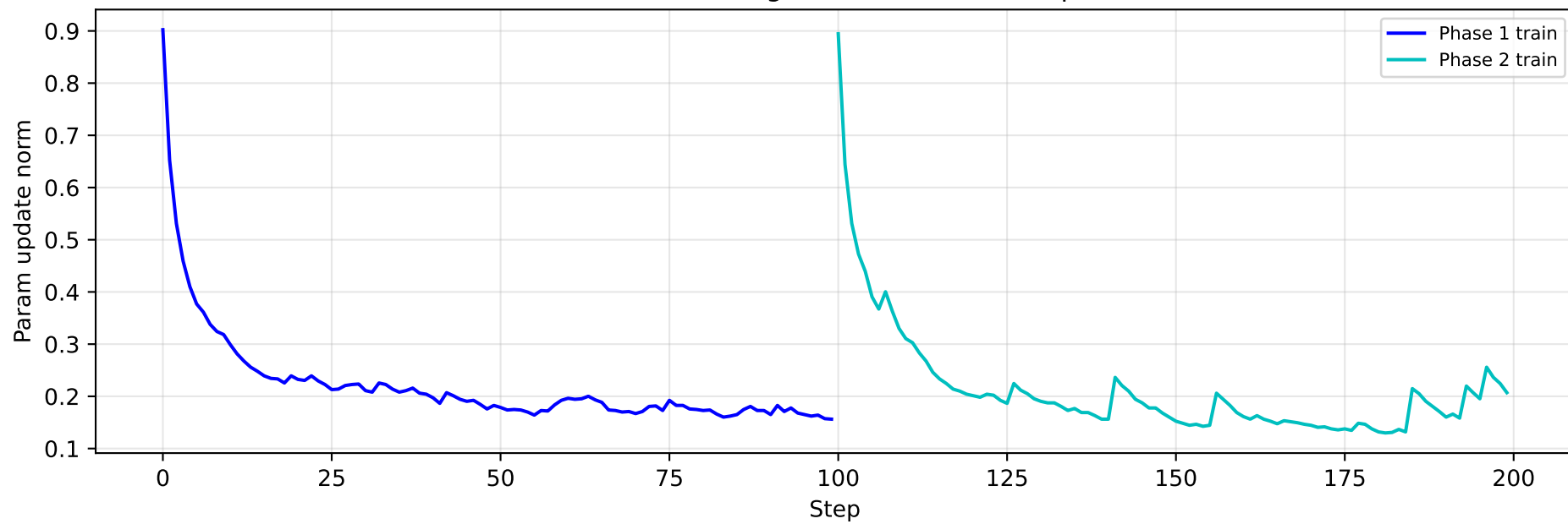
Parameter shift magnitude (L2 norm of updates)
