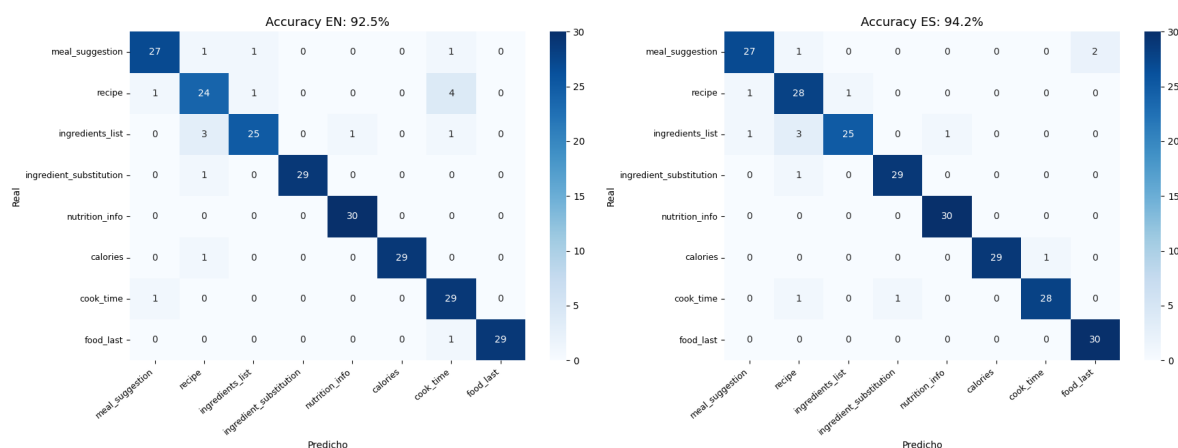
Figura 2: Matrices de confusión por idioma en el conjunto de prueba para T2.
