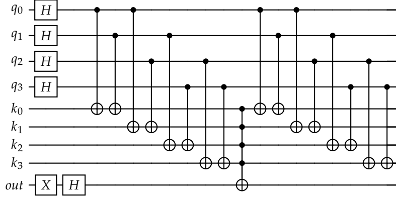
Figura 6.1: Circuito lógico cuántico del oráculo para el problema Sudoku 2 \times 2 . Cuatro qubits lógicos, cuatro qubits ancilla y un qubit output. [37]
