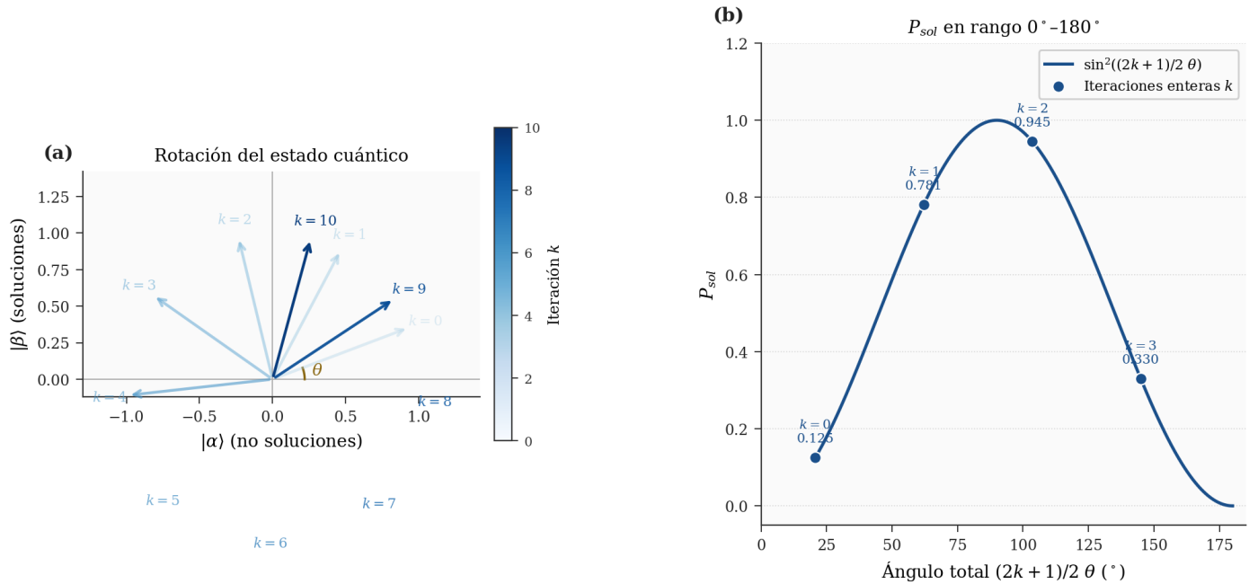
Figura 6.6: Interpretación geométrica de la iteración de Grover para la resolución del Sudoku 2 \times 2 . (a) Rotación del vector de estado en el plano generado por los subespacios de estados solución ( |\beta\rangle ) y no solución ( |\alpha\rangle ), en cada iteración k . (b) Evolución de la probabilidad de éxito P(sol) = \sin^2((2k+1)\theta/2) en función del ángulo recorrido \theta .
