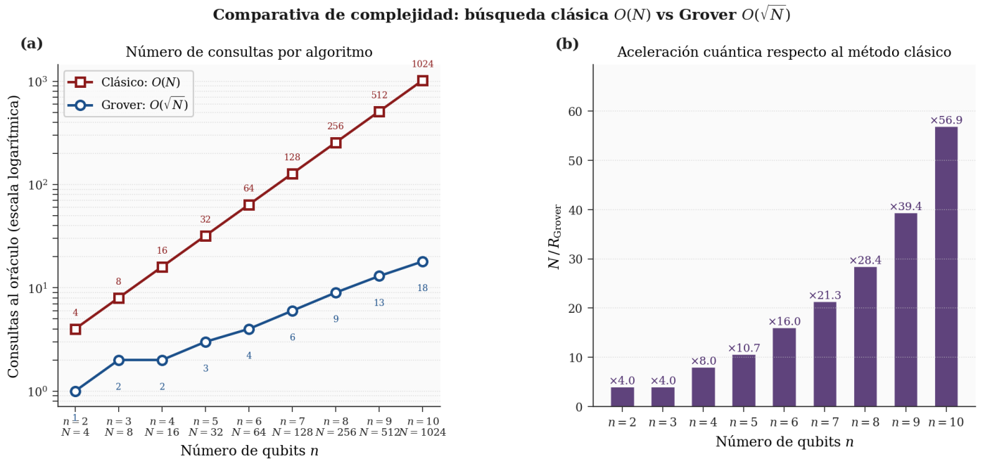
Figura 6.7: Comparativa de la complejidad computacional entre la búsqueda clásica de soluciones, O(N) , y el algoritmo cuántico de Grover, O(\sqrt{N}) , en un espacio de búsqueda de N = 2^n , manteniendo M = 2 constante (a) Consultas al oráculo (escala logarítmica) frente al número de qubits del registro n . (b) Factor de aceleración cuántica, definido como el cociente N/R_{\text{Grover}} .
