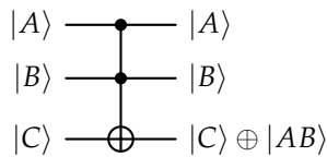
Figura 3.4: Circuito para la puerta de Toffoli.
