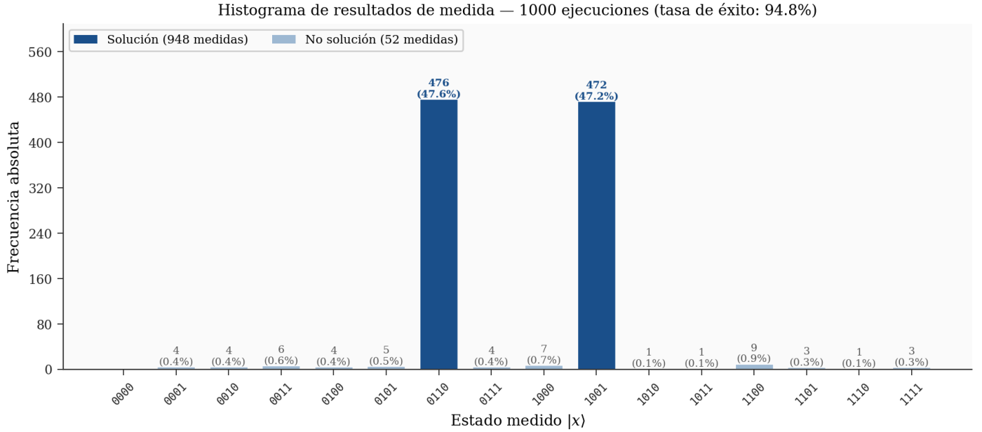
Figura 6.5: Histograma de frecuencias con los resultados de medida tras 1000 ejecuciones independientes del operador de Grover para la resolución del Sudoku 2 \times 2 sobre un circuito de 4 qubits. Estados solución en oscuro y los no solución en claro, con la frecuencia absoluta y el porcentaje correspondiente indicados sobre cada barra.
