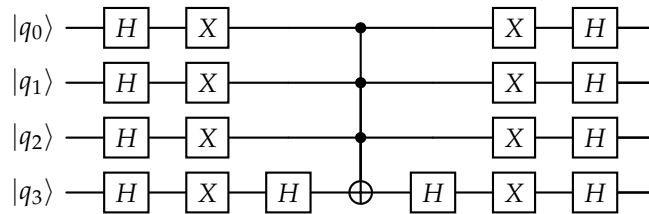
Figura 6.2: Circuito cuántico con 4 qubits para la implementación del operador de difusión, 2|\psi\rangle\langle\psi| - \hat{I} [37].
