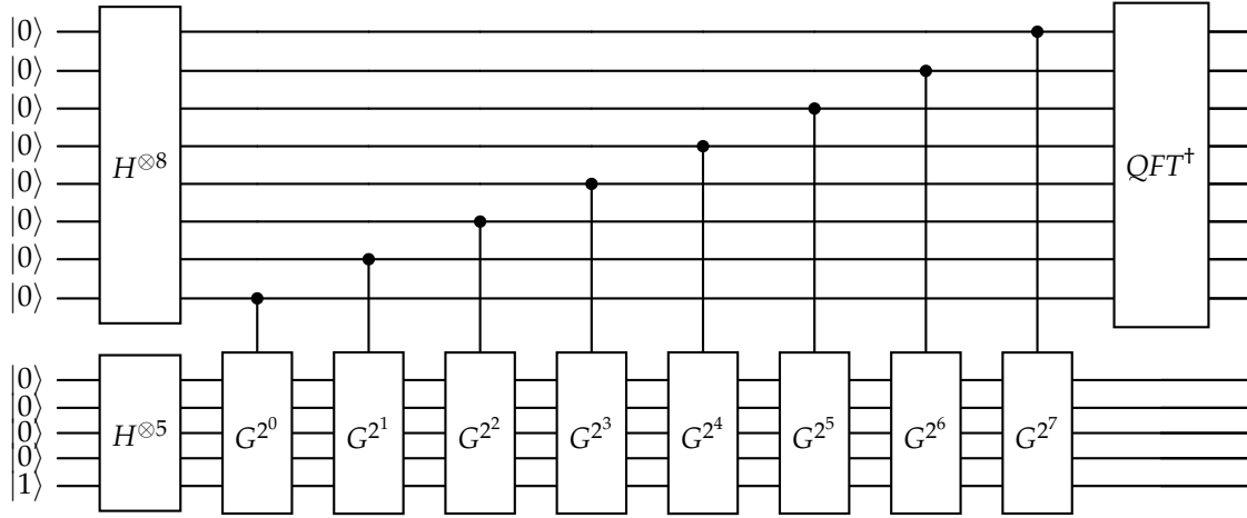
Figura 6.3: Circuito cuántico para la ejecución del conteo cuántico con un operador de Grover previamente diseñado [8].
