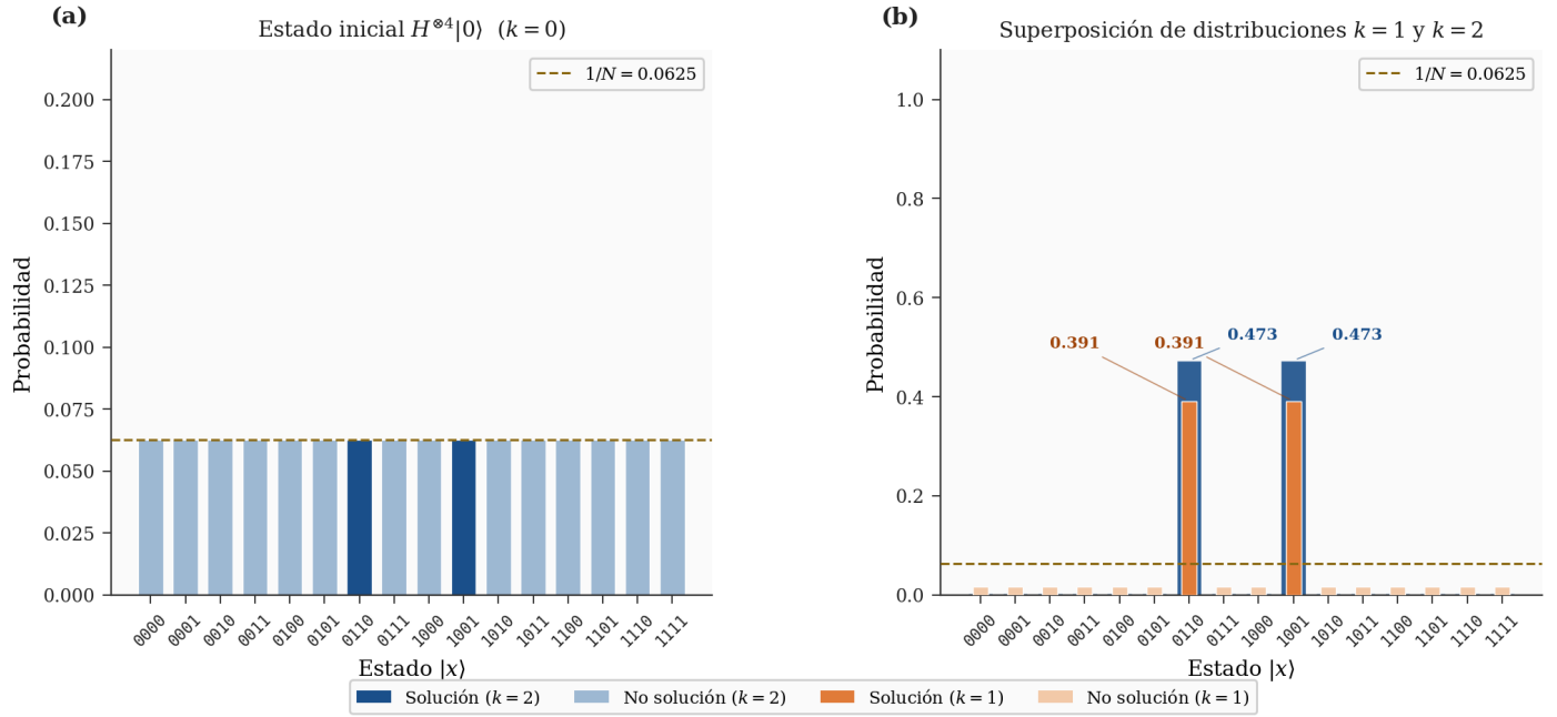
Figura 6.4: Distribuciones de probabilidad de los estados en un circuito de 4 qubits, antes y después de ejecutar el algoritmo de Grover para el Sudoku 2 \times 2 . Estados solución en color oscuro y los no solución en color claro. La línea discontinua marca la probabilidad de los estados en la distribución uniforme. (a) Estado inicial ( H^{\otimes 4}|0\rangle ) equilibrado. (b) Distribuciones superpuestas, en naranja tras k=1 y en azul tras k=R=2 iteraciones de Grover.
