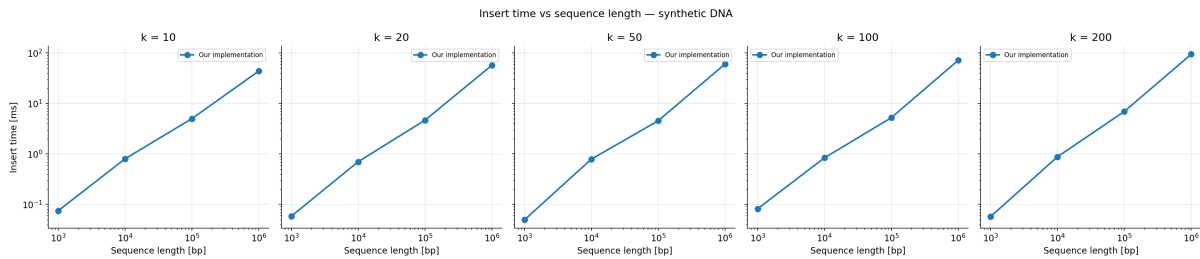
Slika 2: Vrijeme umetanja [ms] u ovisnosti o duljini ulaznog niza [bp] za pet veličina k -mera. Log-log skala. Vrijeme umetanja raste približno linearno s brojem k -mera ( O(n) ), što potvrđuje teorijsku amortiziranu složenost O(1) po umetanju.
