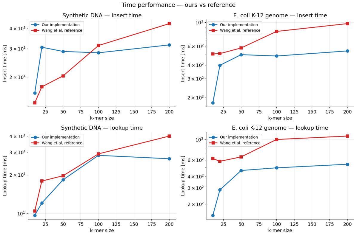
Slika 6: Usporedba vremena umetanja (gore) i pretraživanja (dolje) između naše implementacije (plavo) i referentne (crveno), na sintetičkim podacima (lijevo) i E. coli genomu (desno). Skale su logaritamske; manje je bolje.
