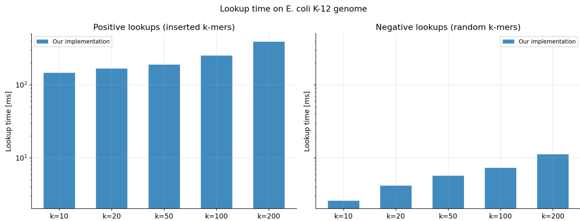
Slika 3: Vrijeme pretraživanja [ms] na genomu E. coli . Pozitivni upiti (lijevo, \sim 4,6 \cdot 10^6 upita) i negativni upiti (desno, 10^5 upita) — skala logaritamska. Negativni upiti su brži za 1–2 reda veličine jer u velikoj većini slučajeva niti jedan otisak u dva kandidatska bucket-a ne odgovara, pa pretraga rano staje.
