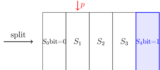
Slika 1: Shematski prikaz operacije dijeljenja segmenta. Otisci iz S_0 redistribuiraju se u S_0 (bit 0 otiska na razini L je 0) i novostvoreni S_4 (bit 0 = 1).
