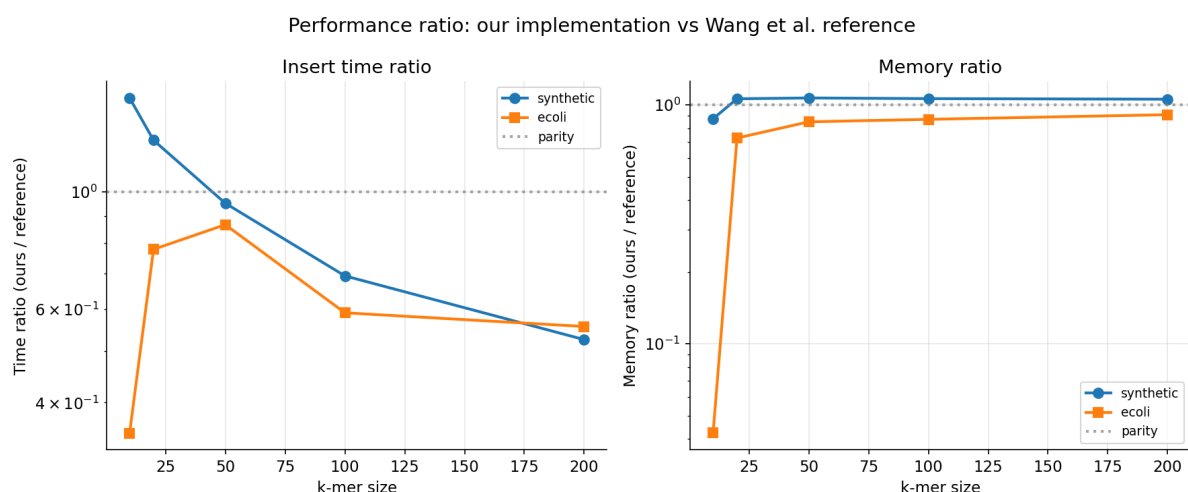
Slika 7: Omjer performansi naše implementacije naspram referentne, u ovisnosti o veličini k -mera. Lijevo: omjer vremena umetanja; desno: omjer zauzeća memorije. Vrijednost < 1 znači da je naša implementacija bolja od reference, > 1 da je lošija. Iscrtana linija označava paritet (1,0). Skale su logaritamske.
