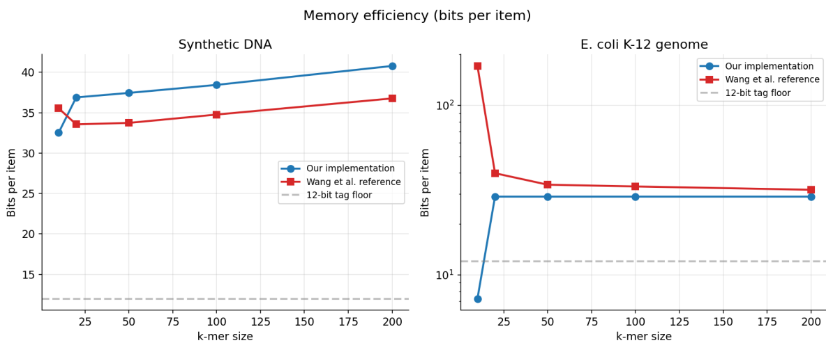
Slika 5: Memorijska efikasnost izražena u bitima po elementu. Plavo: naša implementacija; crveno: referentna implementacija. Iscrtana linija označava teorijski minimum od 12 bita (samo otisak). Desno ( E. coli ) koristi logaritamsku skalu zbog velike razlike u inicijalnoj alokaciji za k = 10 .
