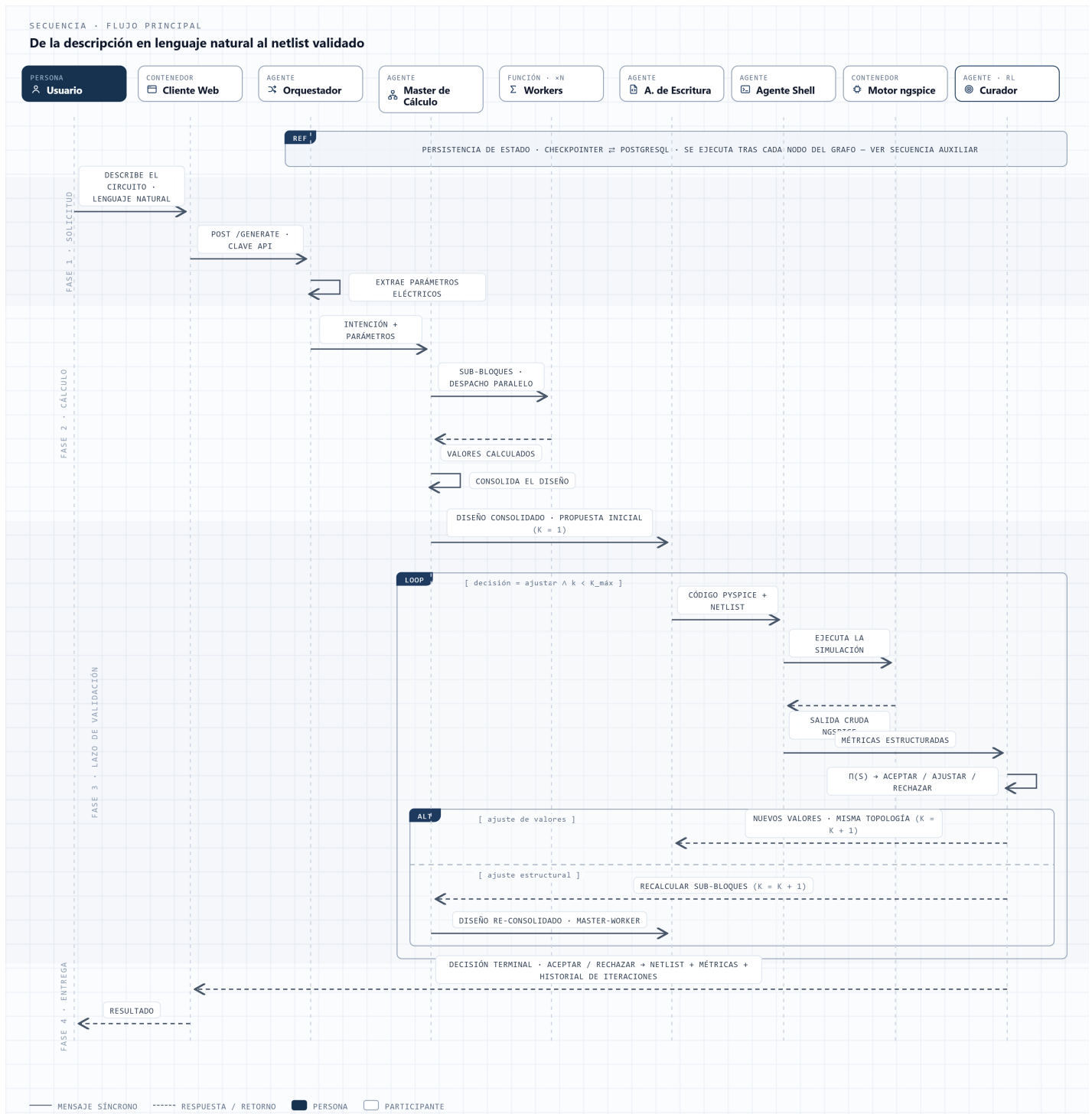
Figura 4.6. Diagrama de secuencia del flujo de generación.
