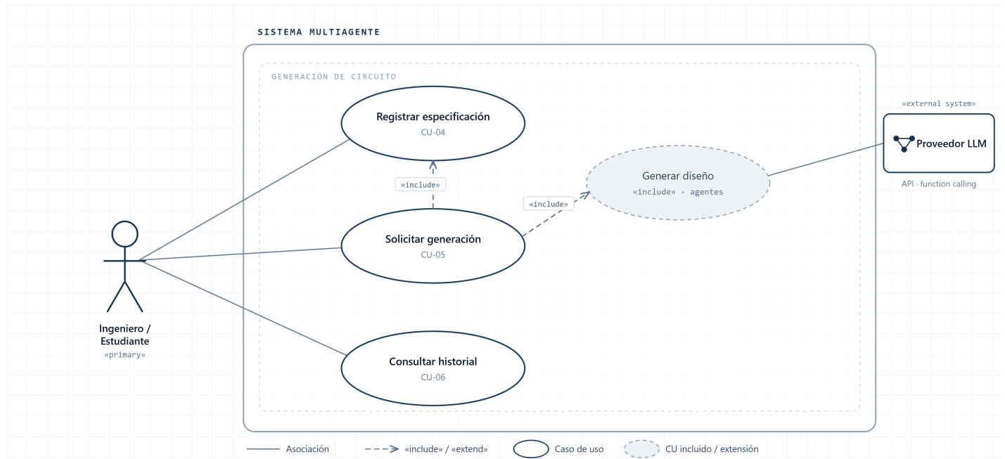
Figura 4.2. Diagrama de casos de uso.
