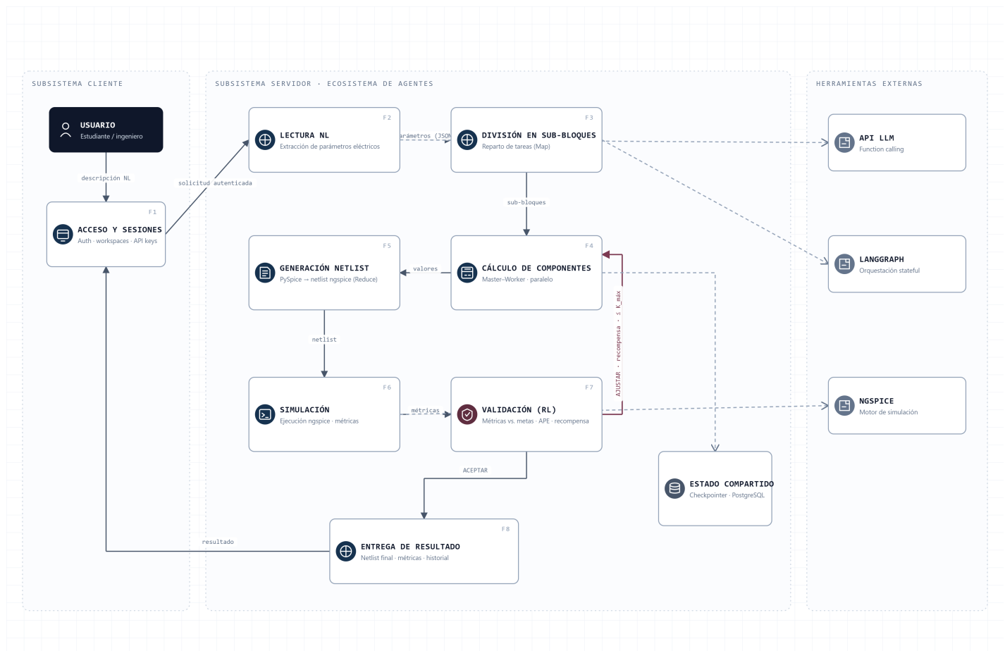
Figura 4.1. Diagrama funcional del sistema.
