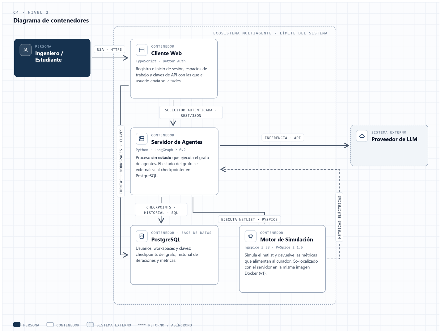
Figura 4.4. C4 Nivel 2: Diagrama de contenedores.
