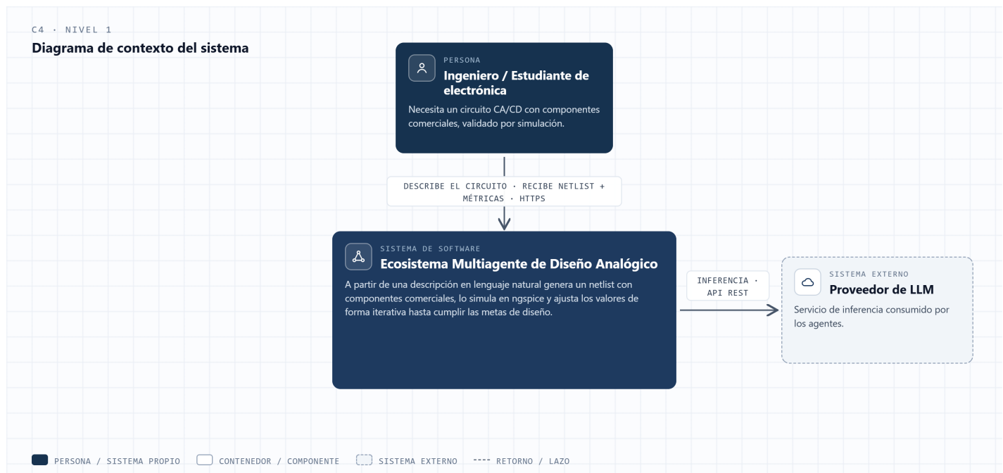
Figura 4.3. C4 Nivel 1: Diagrama de contexto.
