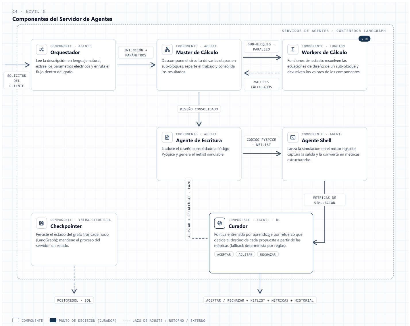
Figura 4.5. C4 Nivel 3: Diagrama de componentes.
