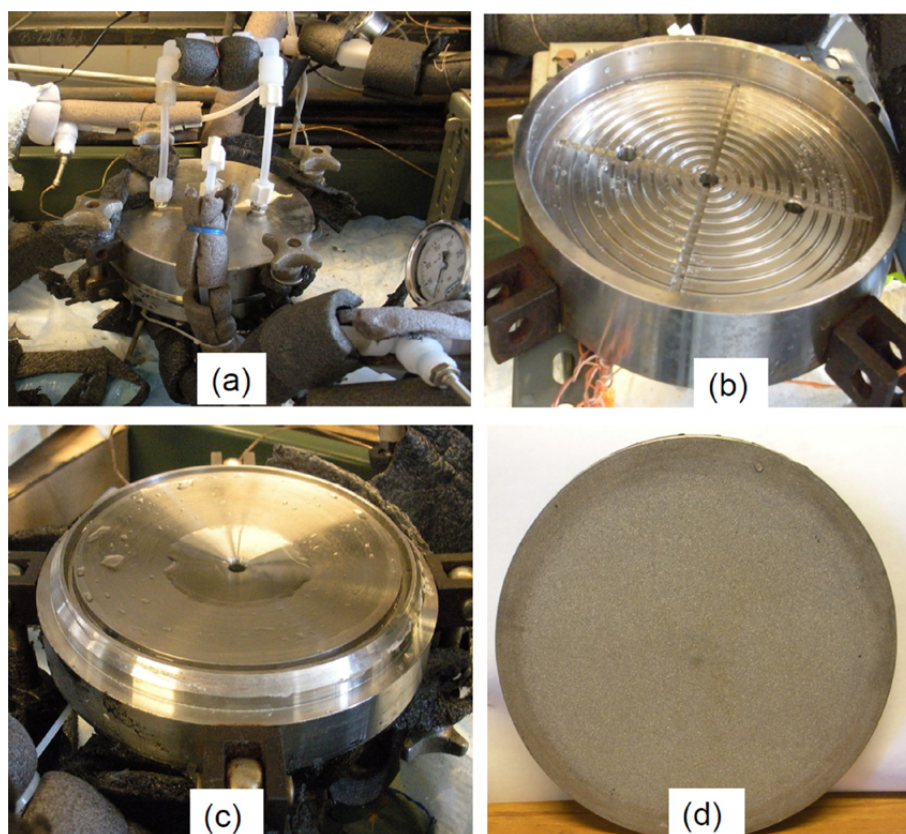
Figura 2.2: Módulo DCMD utilizado no artigo [38]: a) Módulo montado, b) Parte superior do módulo, c) Parte inferior do módulo e d) Suporte da membrana.
