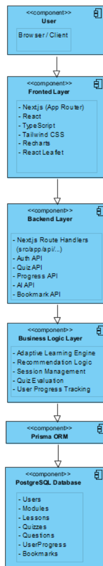
Σχήμα 2: Architecture Diagram
