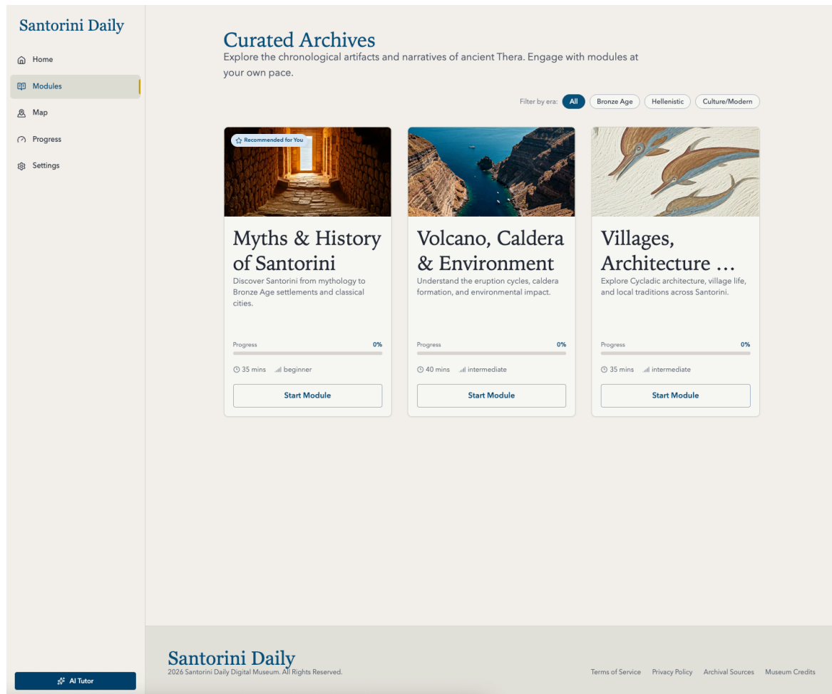
Σχήμα 6: Modules menu
