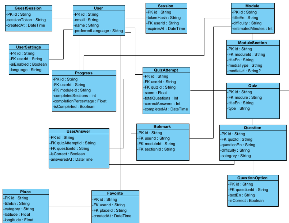
Σχήμα 4: Διάγραμμα βάσης
