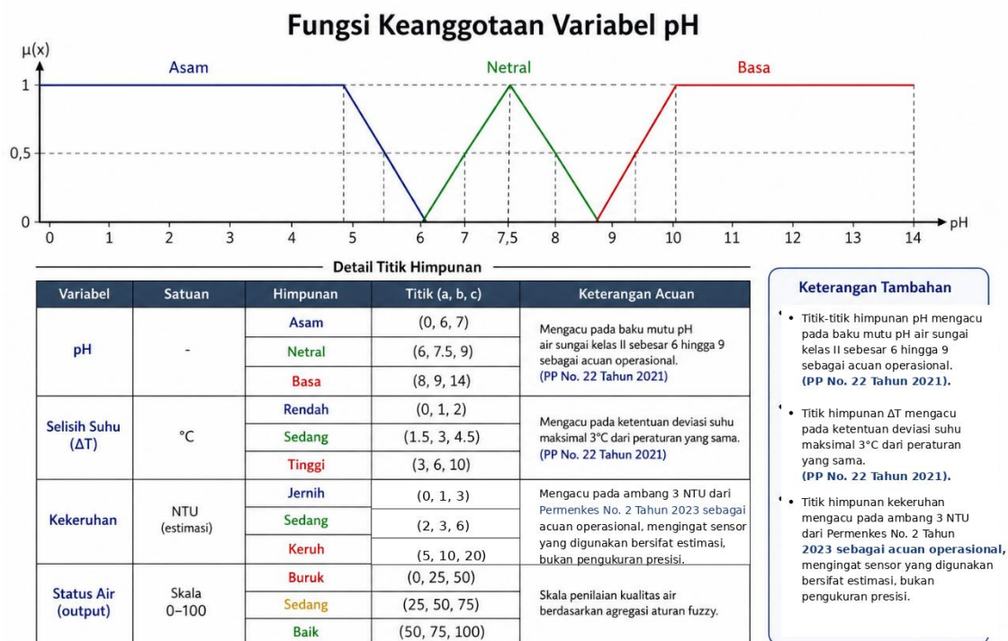
Gambar 3. 5 Gambar Fungsi Keanggotaan Variabel pH
