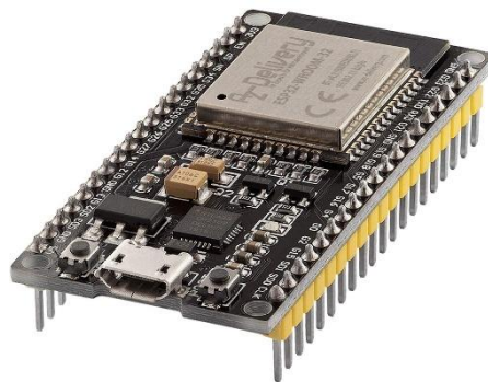
Gambar 2. 1 Modul ESP32 DevKit V1
