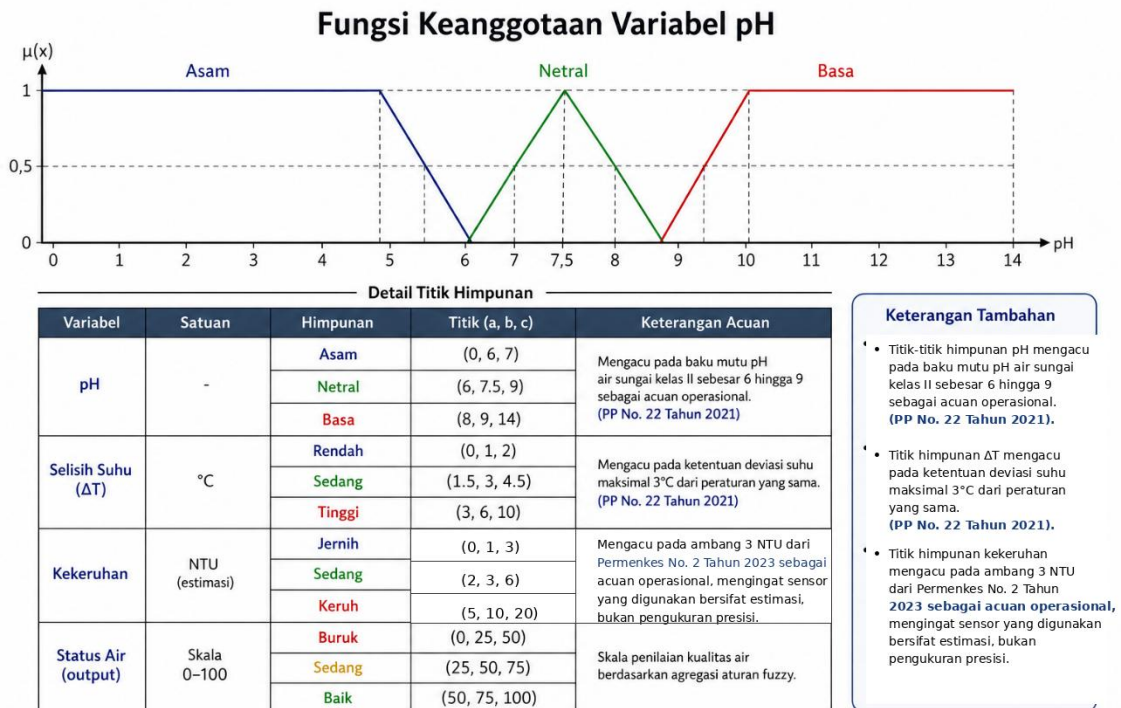
Gambar 3. 4 Gambar Fungsi Keanggotaan Variabel pH
