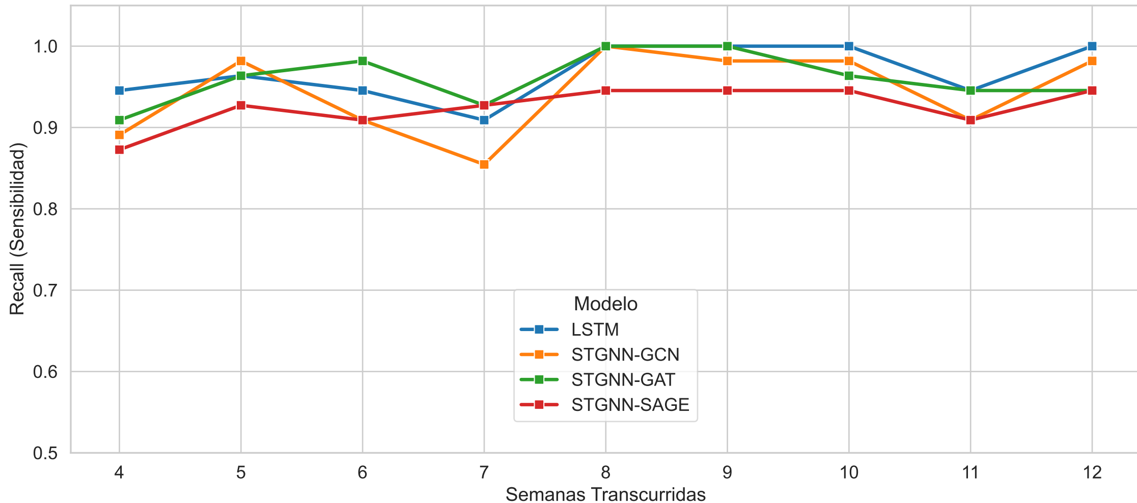
Comparativa de Sensibilidad (Recall) entre Modelos
