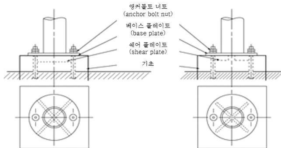
그림 2.2.3.6 구형저장탱크 지주와 기초에 앵커볼트 체결방법
