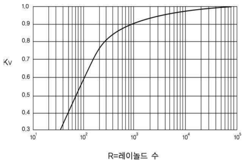
그림 2.8.1.4.2② 점도로 인한 용량보정계수
