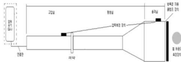
그림 4.2 폭발압력저항시험장치 구성도
