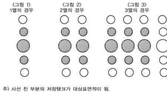
그림 2.9.9.1.4 온도상승방지설비 능력산정기준
