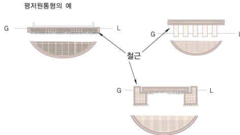
그림 2.2.2.3 저장탱크의 수평기초면
