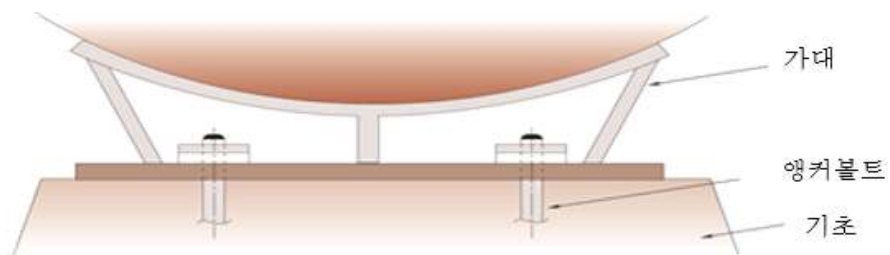
그림 2.2.3.4 앵커볼트의 고정방법 &lt;개정 16. 12. 15&gt;
