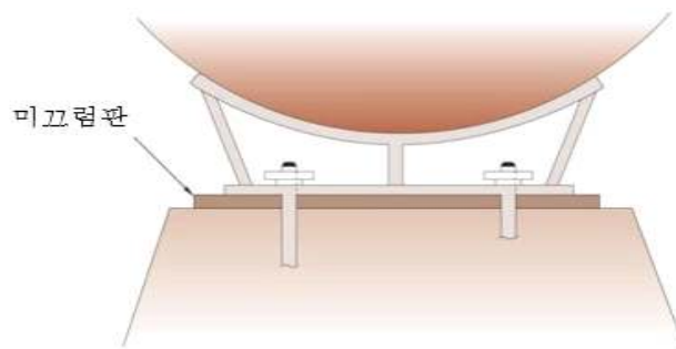
그림 2.2.3.5 미끄럼판의 설치방법
