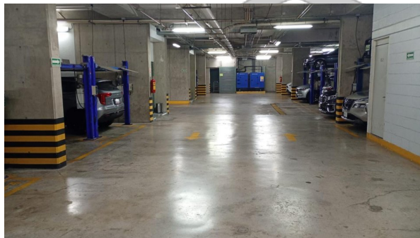
Foto 15. Estacionamiento – plataformas y cuarto de equipos
