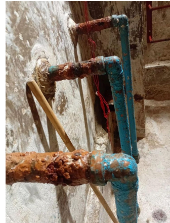
Tuberías de alimentación con corrosión severa.
