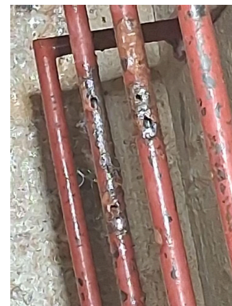
Escalera marina con corrosión y perforaciones (retirada).
