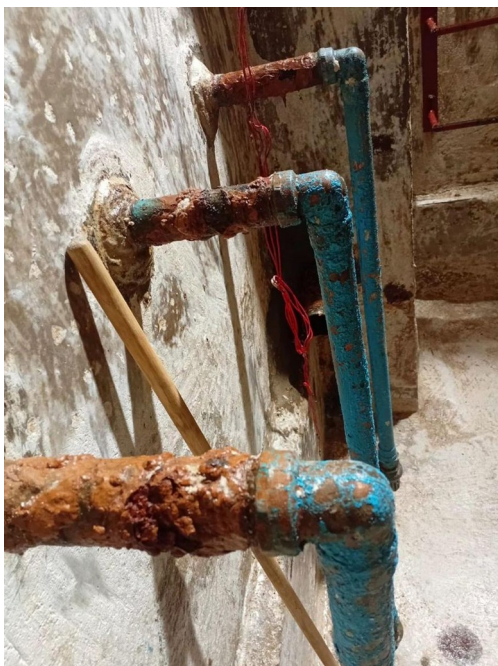
Tuberías de succión con corrosión severa (antes; detectado por el Comité).
