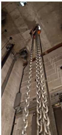
Cabina asegurada con polipasto de cadena en el cubo del elevador.
