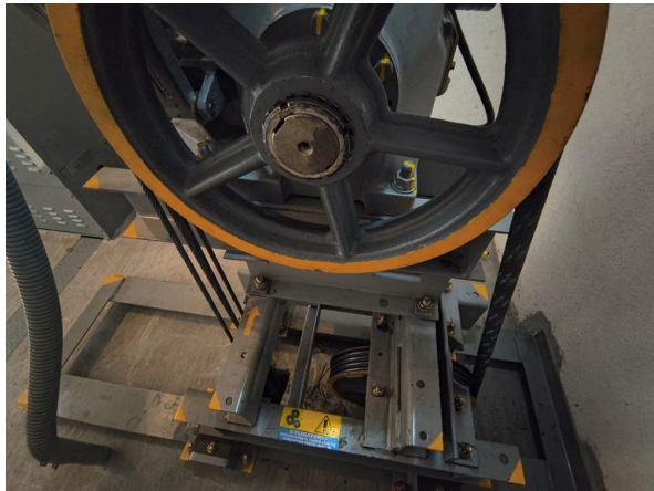
Cables nuevos hacia la polea deflectora.
