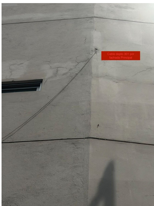
Fachada principal: cable del Depto. 301 fijado por fuera, con perforación en el muro y grietas alrededor.
