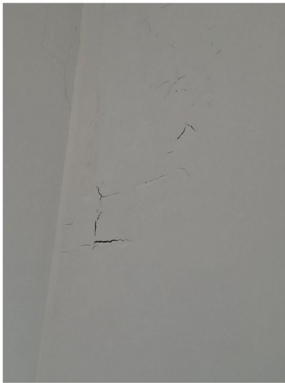
Vista exterior — detalle del cuarteamiento superficial del aplanado. El patrón confirma deterioro por saturación interna.
