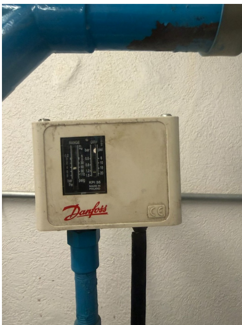
Presostato del sistema hidroneumático revisado durante la evaluación de equipos.
