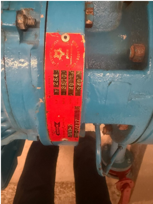
Placa de datos de la bomba, registrada por el Comité para el expediente técnico de los equipos.
