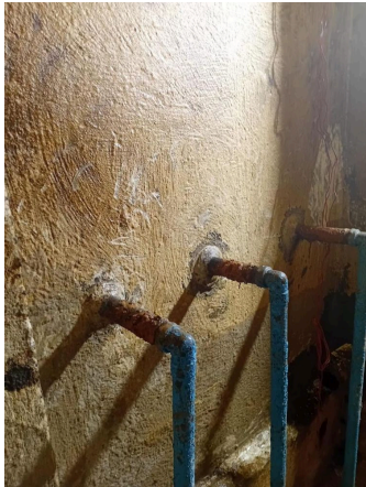
Muros con impermeabilizante deteriorado y tuberías oxidadas.
