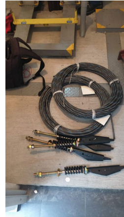
Cables nuevos y 4 tensores de resorte para amarre.
