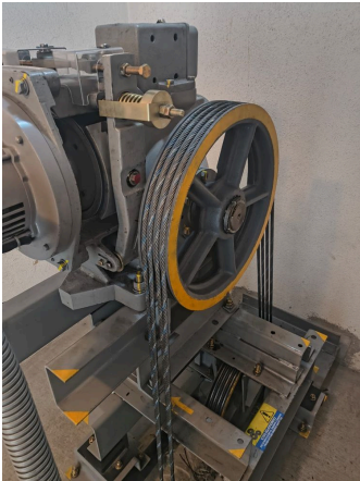
Cables nuevos montados en la polea de tracción.
