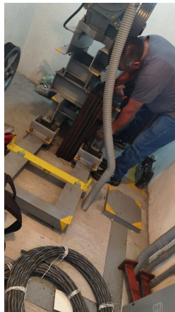
Instalación de cables nuevos a través de la losa.
