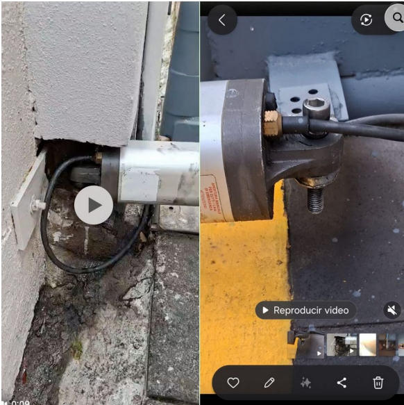
Brazo hidráulico del portón y su soporte de sujeción.
