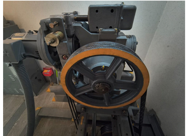
Máquina de tracción con cables nuevos, vista frontal.
