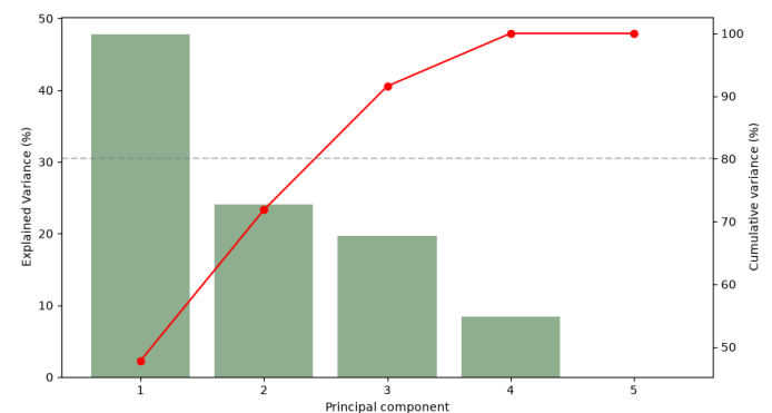
Figura 4. Scree plot delle componenti principali — LL globale (sintetico).
