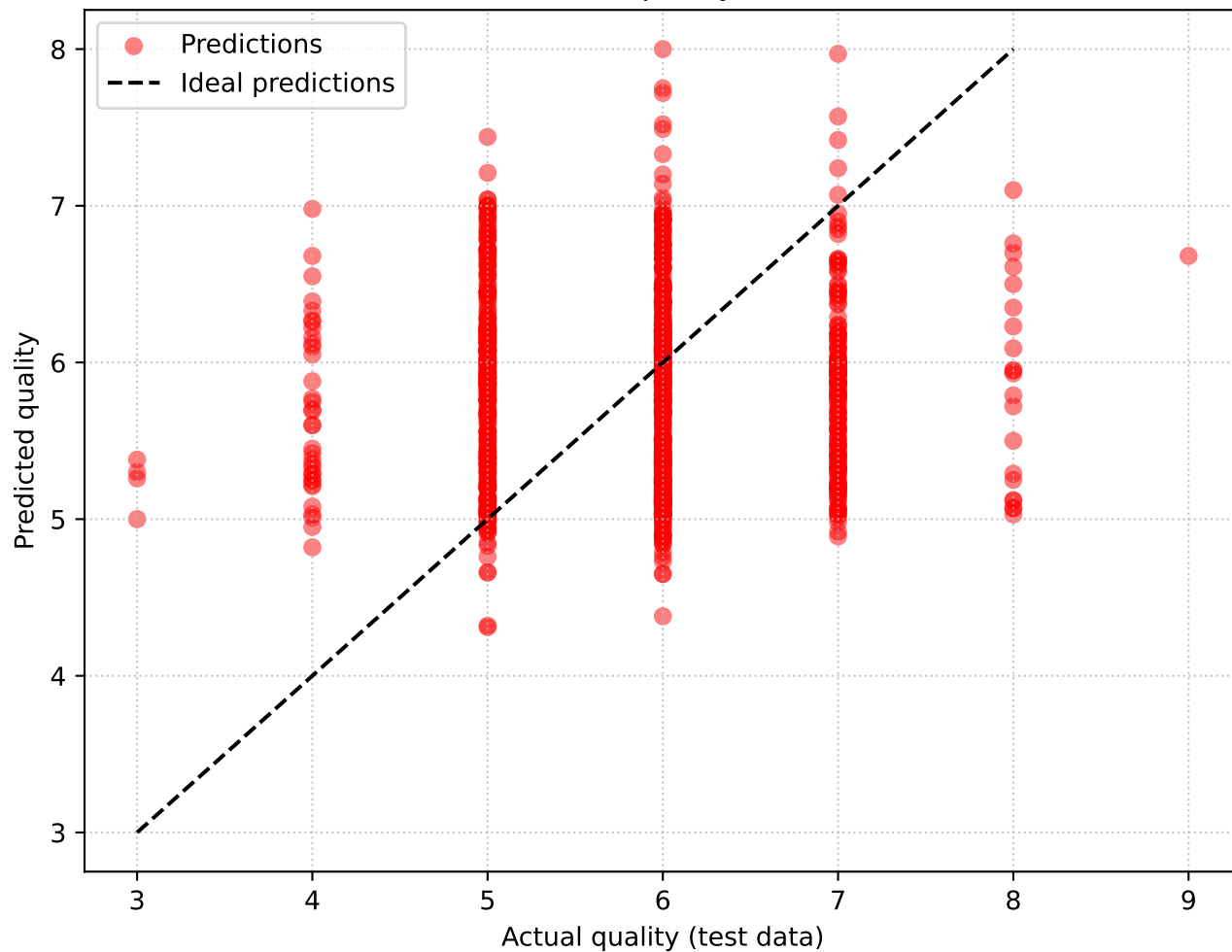
Predicted vs actual quality - Random Forest
