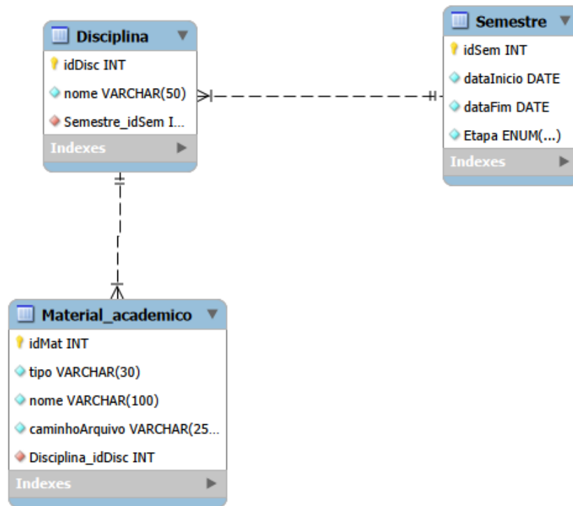
Figura 2: Projeto Lógico (EER) do sistema.
