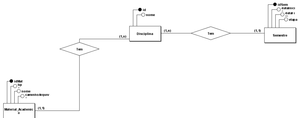
Figura 1: Diagrama Entidade-Relacionamento (DER) do sistema.
