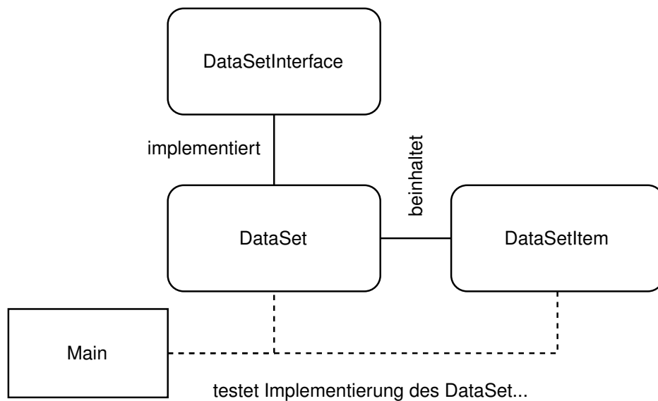
Abbildung 1: Klassendiagramm
