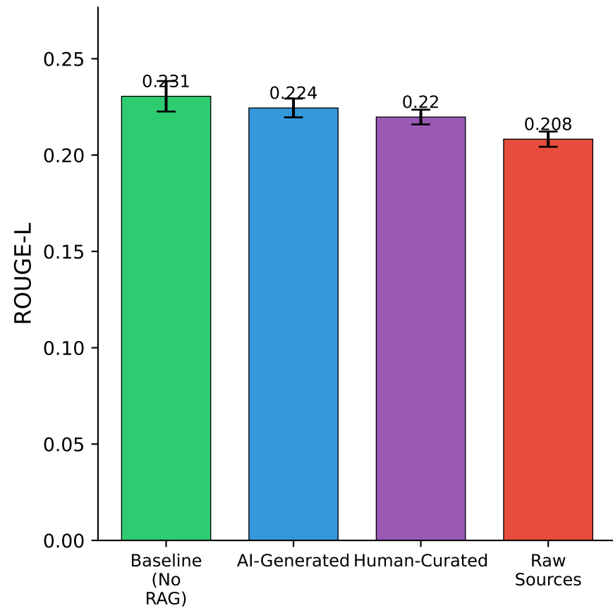
ROUGE-L
