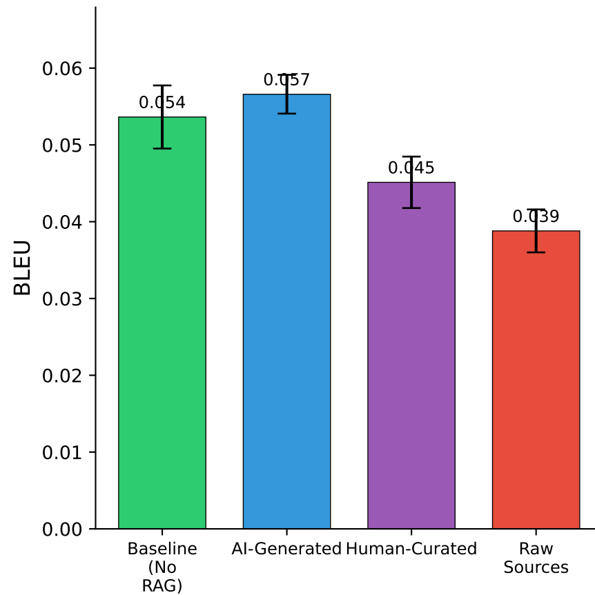
BLEU
