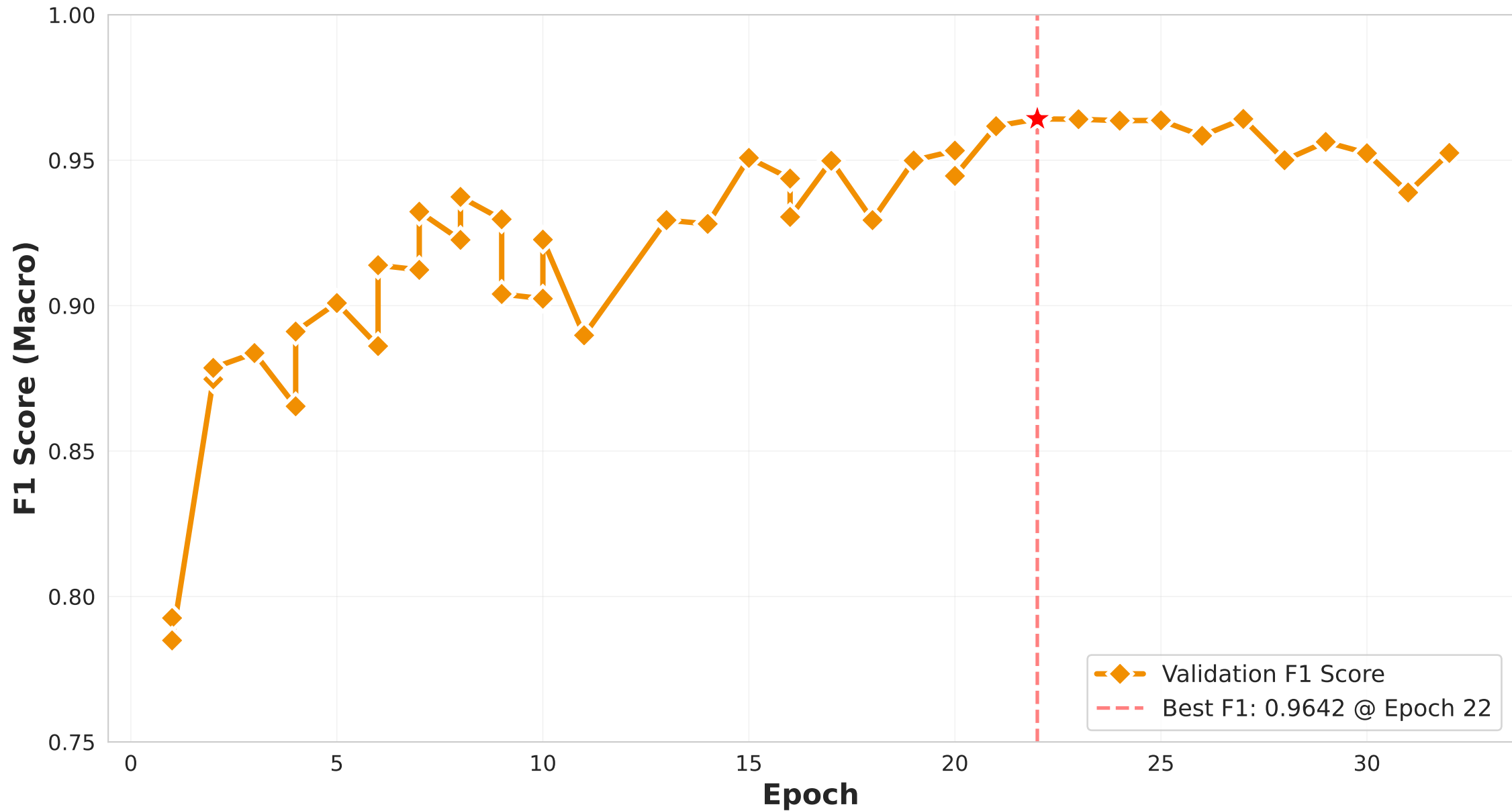
Validation F1 Score Over Epochs
