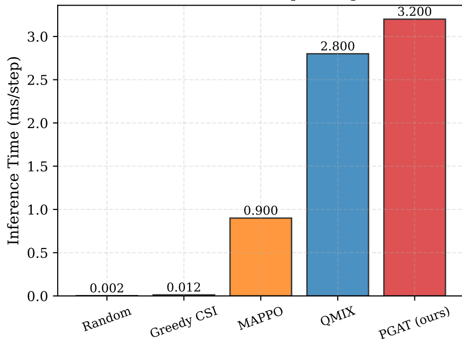
Inference Time per Step
