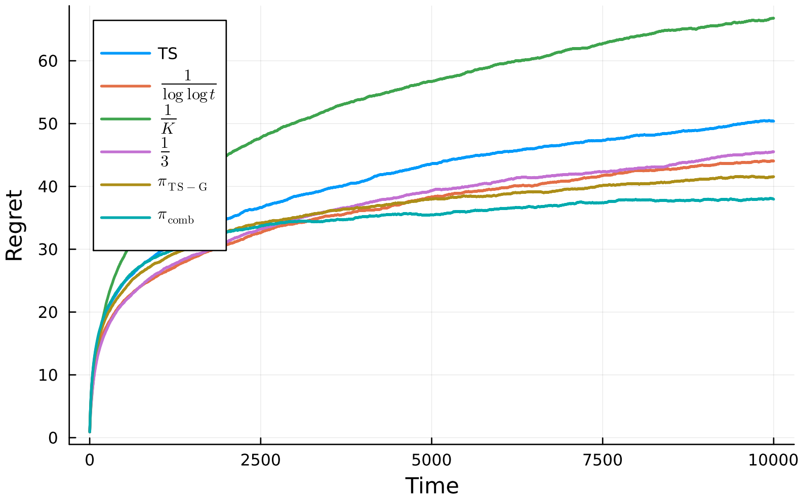
Regret avg. over 1 runs, 10 arms (Bernoulli)
