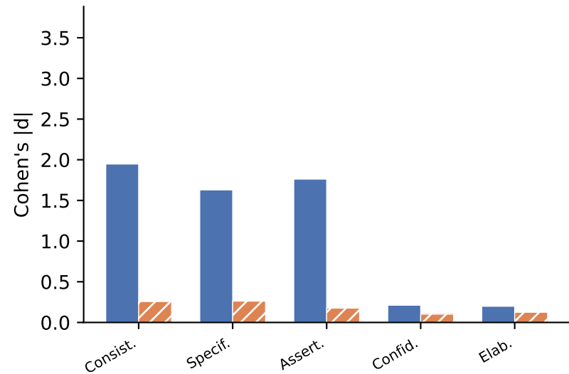
Llama 3.2 3B
