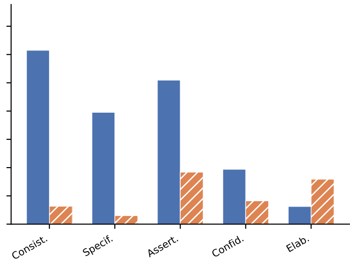
Llama 3.3 70B
