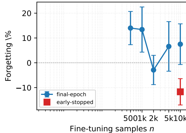
(d) Task forgetting
