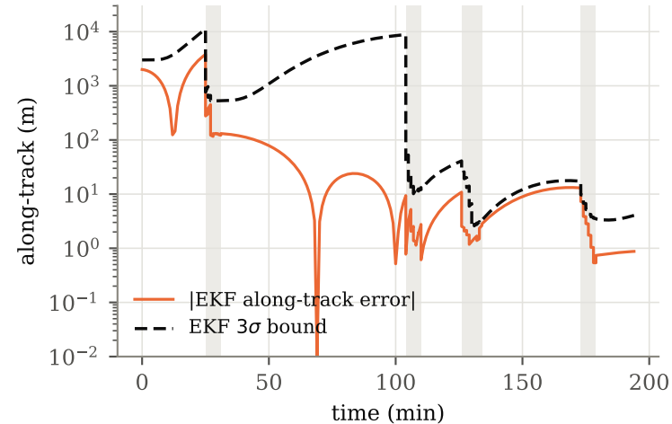
(a) EKF
