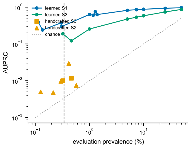
(b) AUPRC
