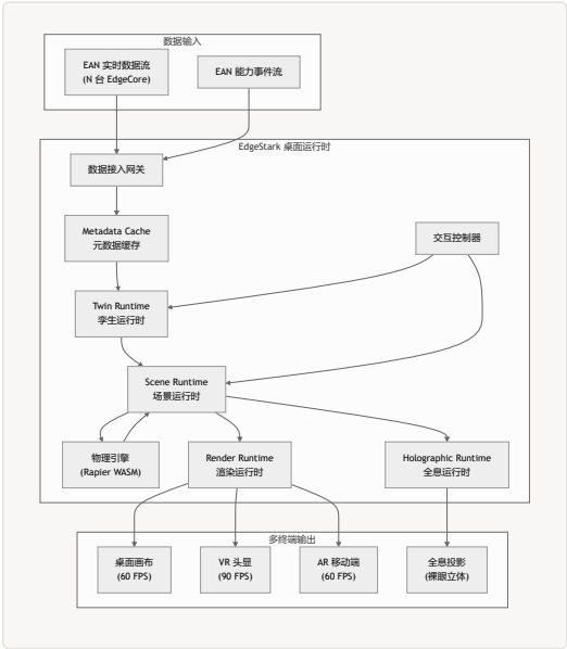
图 3 EdgeStark 内部架构：五运行时协作与四终端输出
