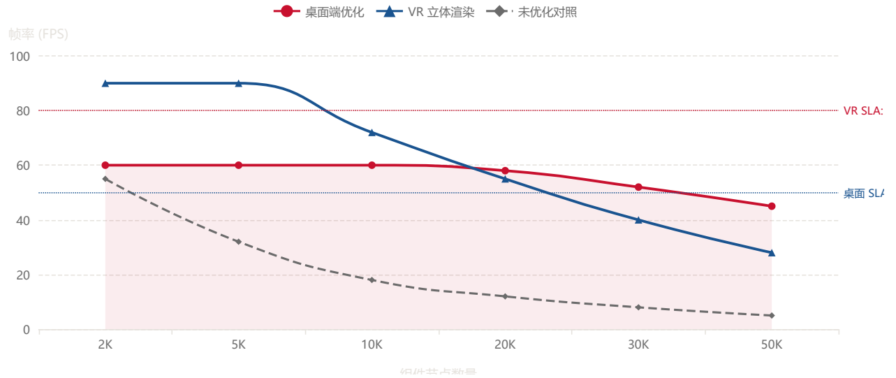
图 11 三维渲染帧率 vs 场景复杂度 (桌面端与 VR 立体渲染)
