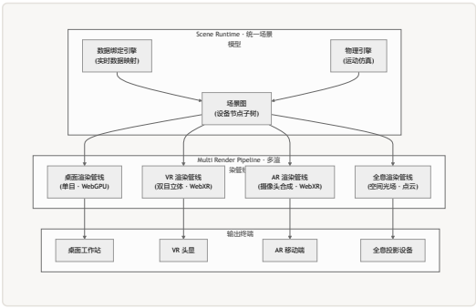
图 5 统一场景模型与多渲染管线架构
