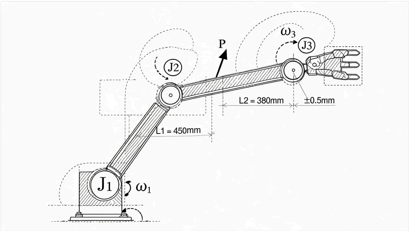
图 8 实时物理仿真示意：机械臂运动学仿真、碰撞检测区域与刚体约束系统
