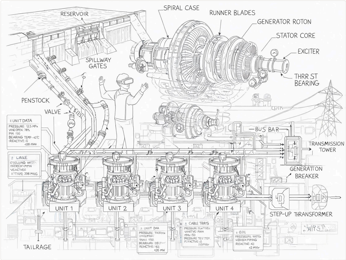
图 24 水电站数字孪生场景：水轮发电机组三维模型与实时运行参数全息叠加
