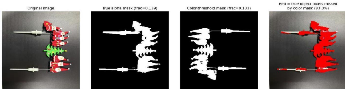
Hình 6: FA-1047, một mẫu bình thường. Từ trái sang phải, ảnh gốc; mặt nạ alpha thực (phân đoạn mới). đầu ra mô hình); mặt nạ ngưỡng màu (từ tập dữ liệu đã loại bỏ nền); các pixel hiện có trong Mặt nạ thật nhưng bị mặt nạ ngưỡng màu bỏ sót, được tô đỏ. Mặt nạ ngưỡng màu Bỏ sót hầu hết phần để tối màu.
