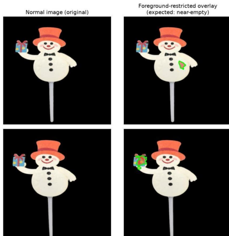
Hình 10: FA-808, các mẫu bình thường được giữ lại ở độ phân giải 384 \times 384 , ngưỡng giới hạn vùng tiền cảnh với mặt nạ đối tượng alpha thực. Các vùng nhỏ riêng lẻ (ví dụ: cạnh của hộp quà) đôi khi được giữ lại, nhưng không tạo ra vùng dương tính giả lớn nào.
