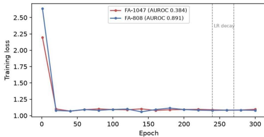
Hình 13: Hàm mất mát huấn luyện cho lần chạy SuperSimpleNet cuối cùng (đã hiệu chỉnh kiến trúc), FA-1047 và FA-808. Hàm mất mát giảm mạnh từ khởi tạo ngẫu nhiên nhưng đạt mức ổn định ở khoảng epoch 20 và không giảm đáng kể trong 280 epoch còn lại, kể cả sau khi tốc độ học giảm dần theo lịch trình ở epoch 240 và 270.
