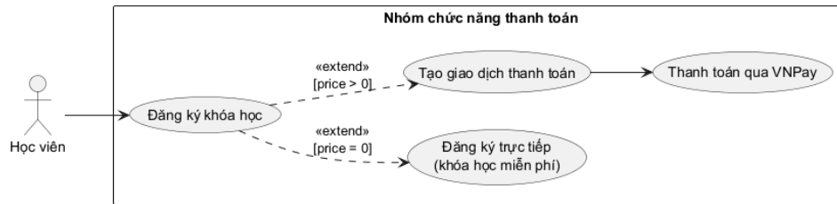
Hình 2.3: Biểu đồ use case phân rõ nhóm chức năng thanh toán
