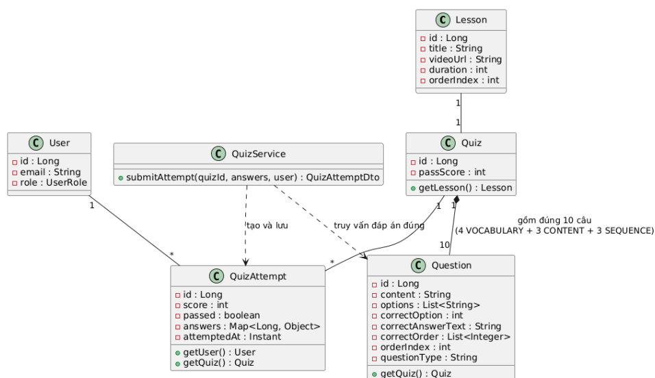
Hình 4.3: Biểu đồ lớp nhóm Quiz
