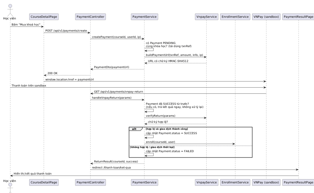
Hình 4.6: Biểu đồ trình tự: Đăng ký khóa học có phí qua VNPAY
