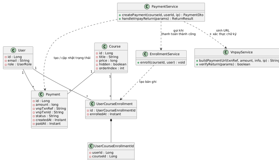
Hình 4.4: Biểu đồ lớp nhóm Enrollment và Payment
