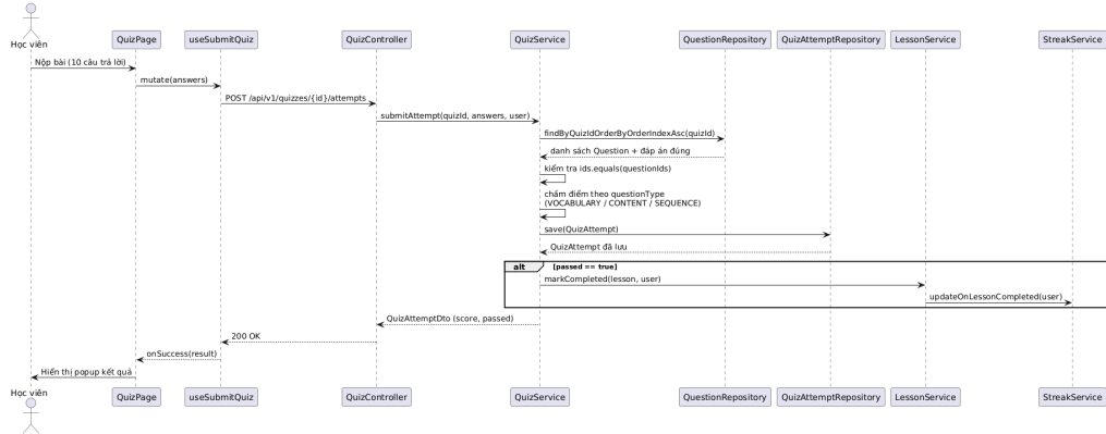
Hình 4.5: Biểu đồ trình tự: Nộp bài quiz
