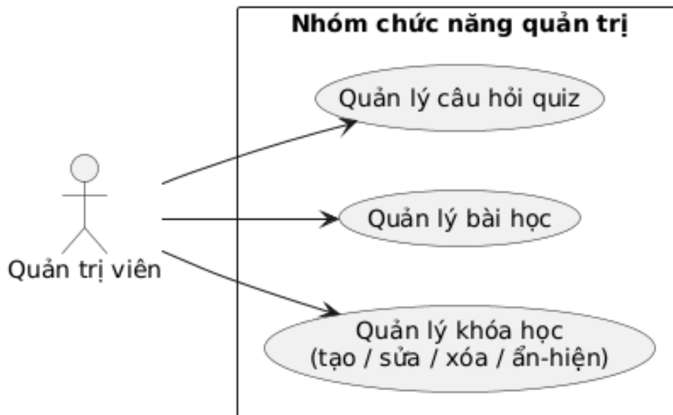
Hình 2.4: Biểu đồ use case phân rõ nhóm chức năng quản trị
