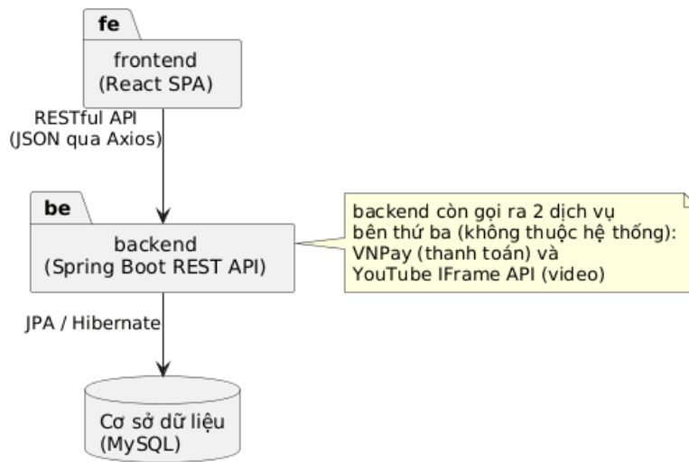
Hình 4.1: Biểu đồ gói tổng quan hệ thống NihongoFlow
