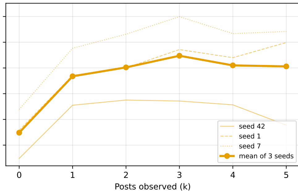
Macro F1
