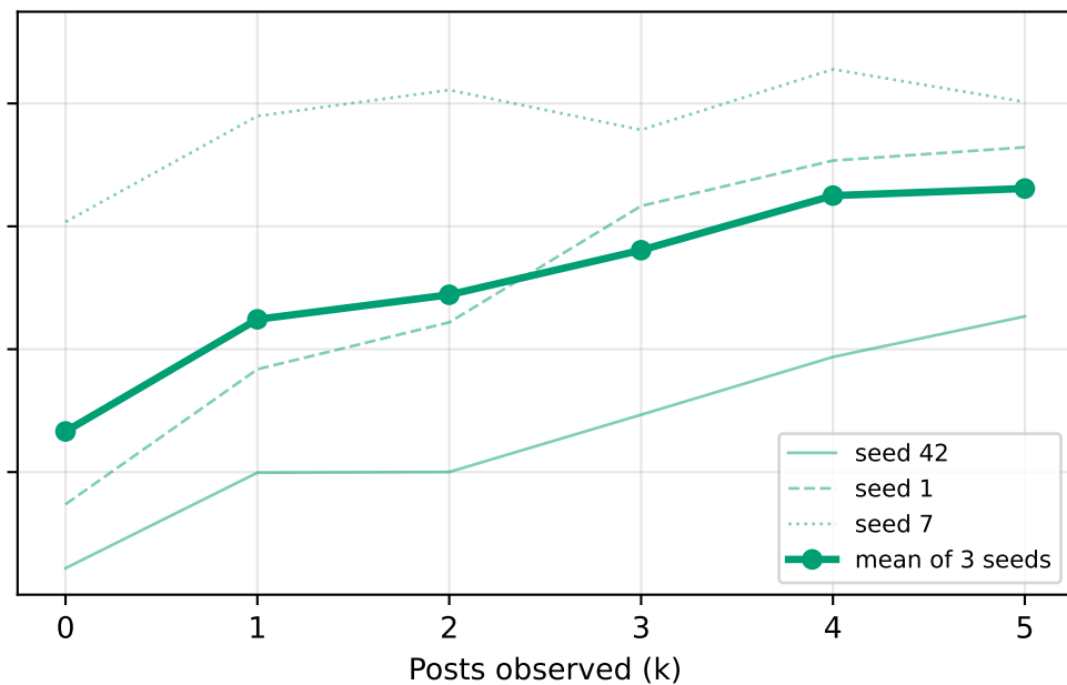
Macro F1
