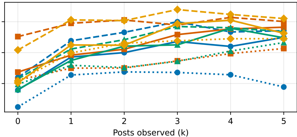
Macro F1
