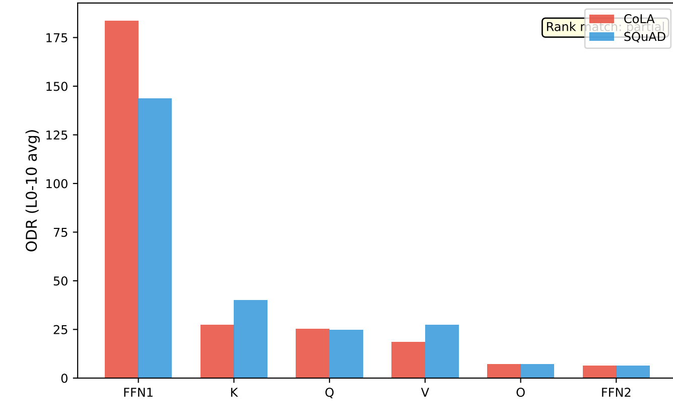
(d) Output Distortion Ratio
