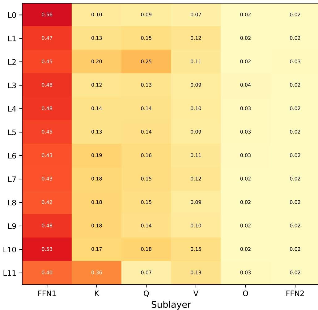
CoLA
