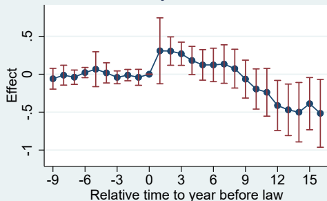
Callaway & Sant'Anna
