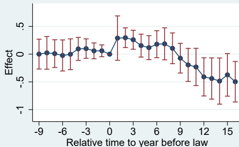
Sun & Abraham
