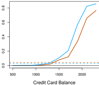
Default Rate
