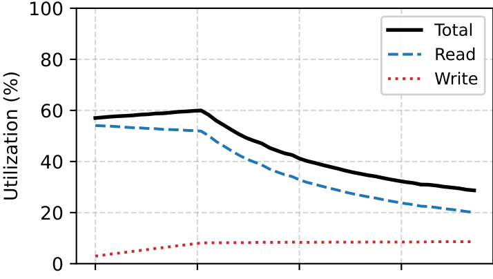
768-Prefill
