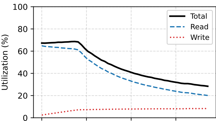
512-Prefill
