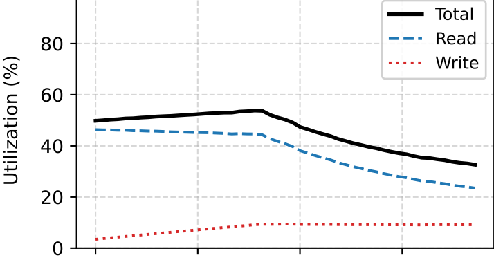
1280-Prefill
