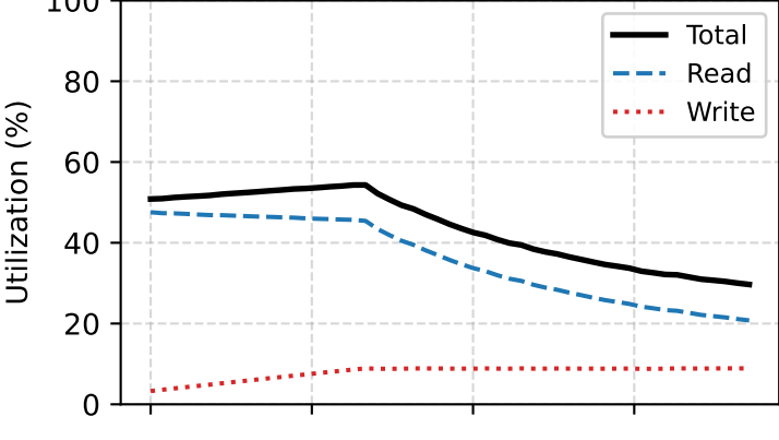
1024-Prefill
