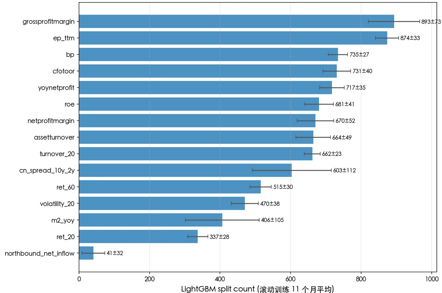
LightGBM 特征重要性 (2024-2025 沪深300 真实数据)
