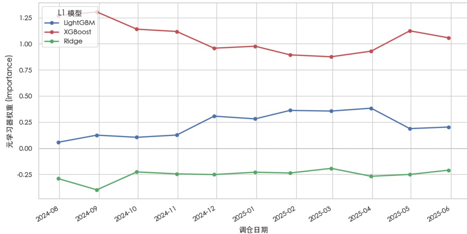
C2 一元学习器 (Ridge) 对 L1 模型权重的滚动估计
