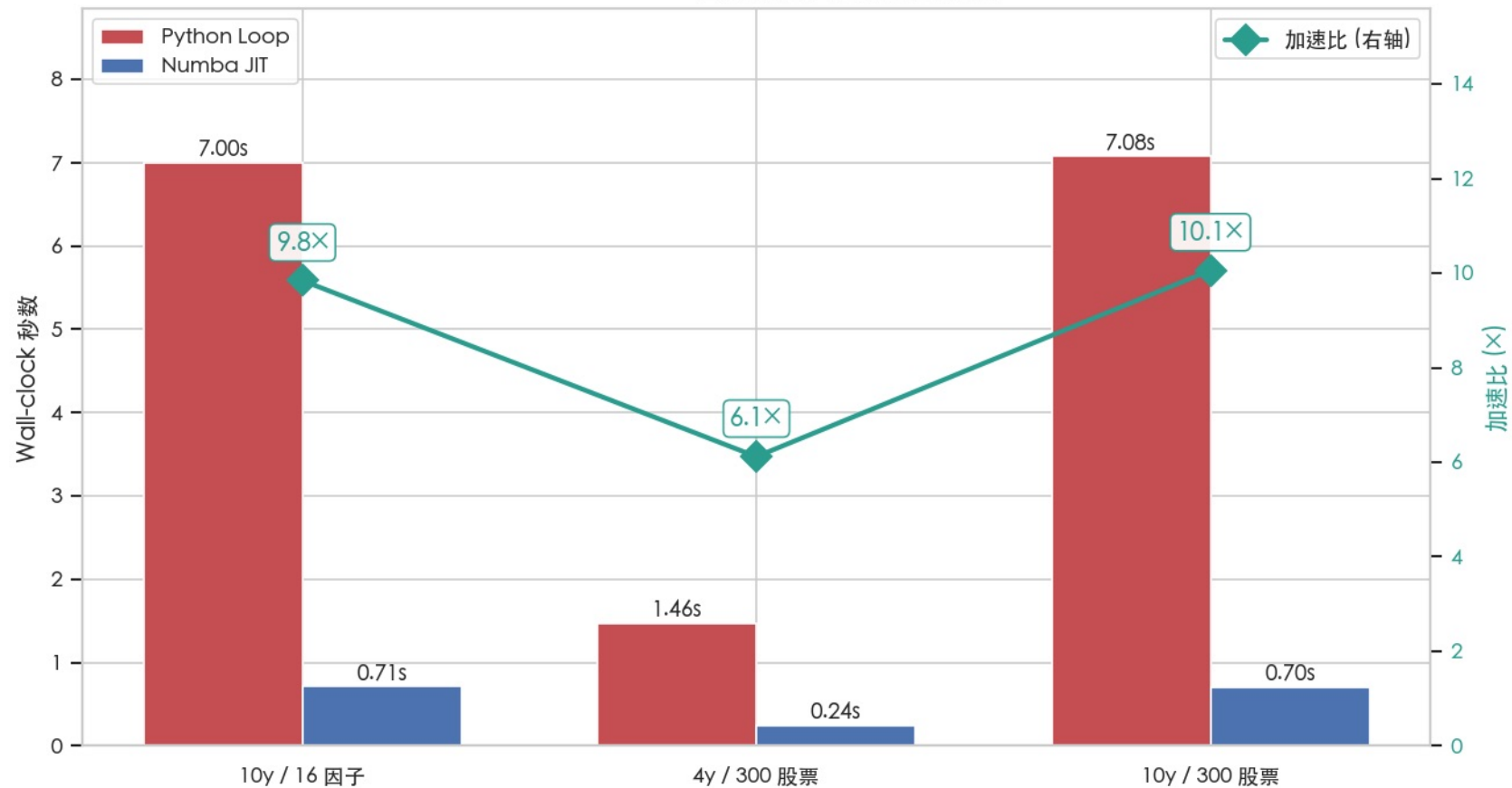
C4 — Numba JIT 回测引擎在不同规模上的加速
