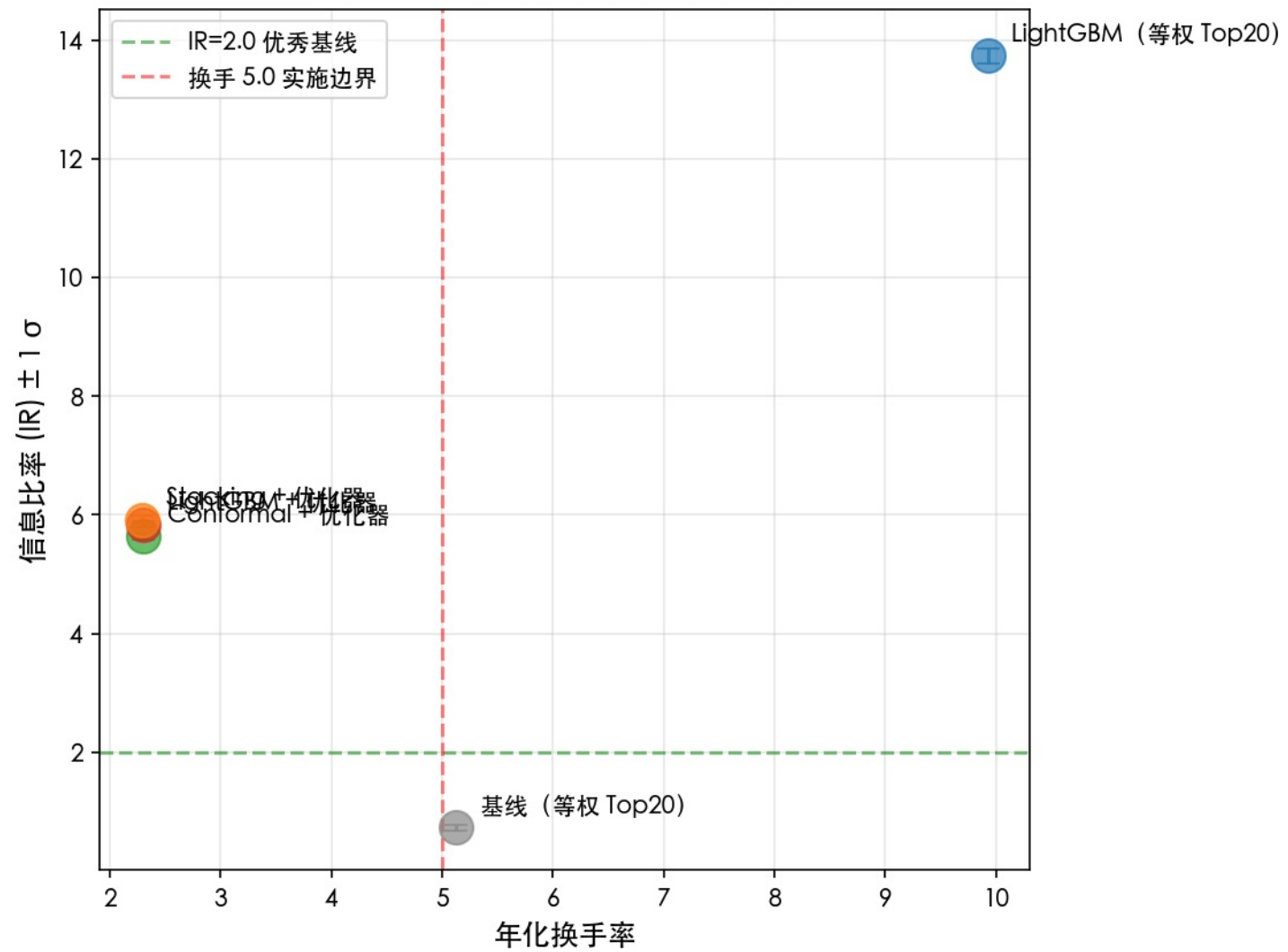
IR vs 换手率 (指数增强可投资性视角)
