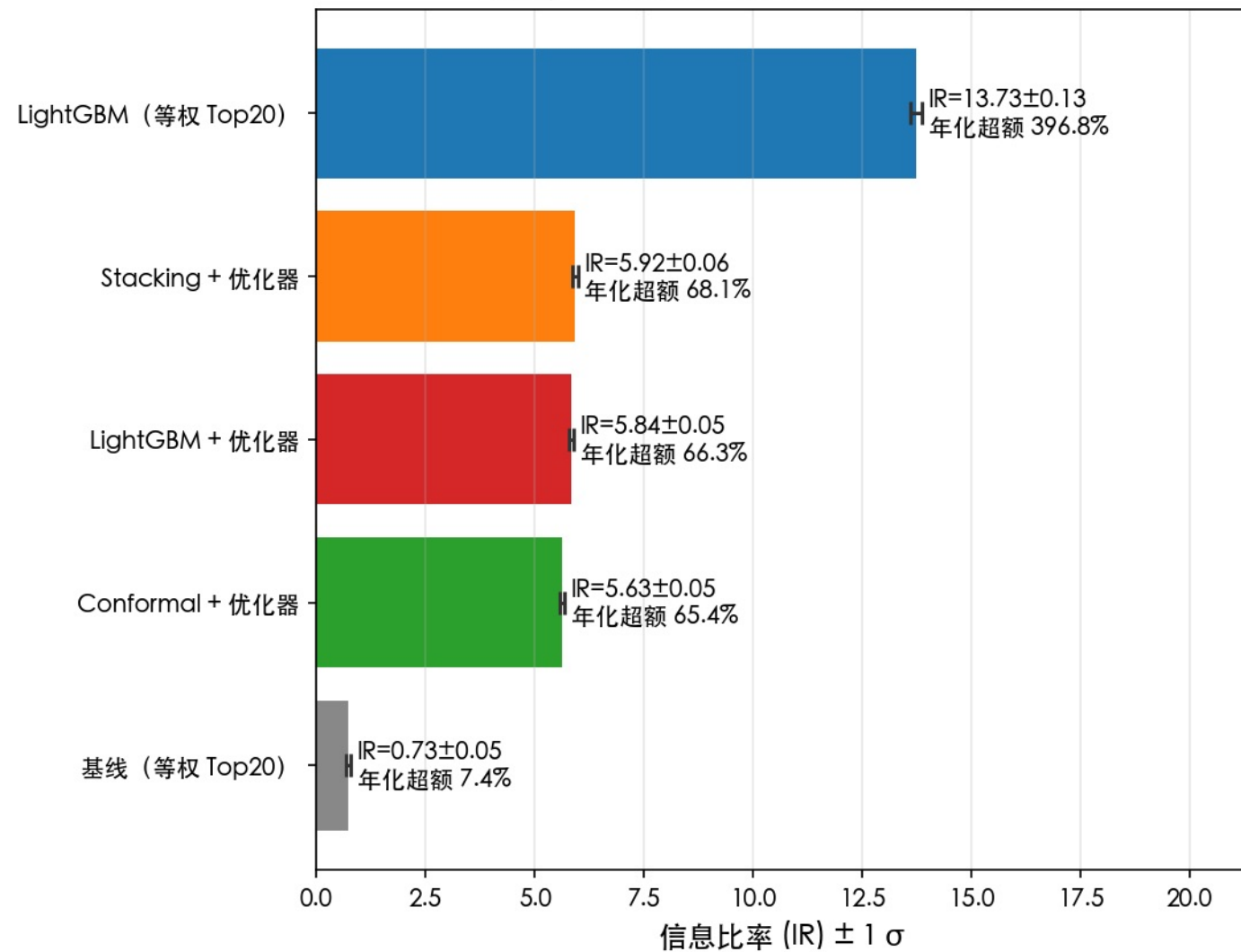
五策略 IR 横向对比 (含 5-seed 不确定性度量)
