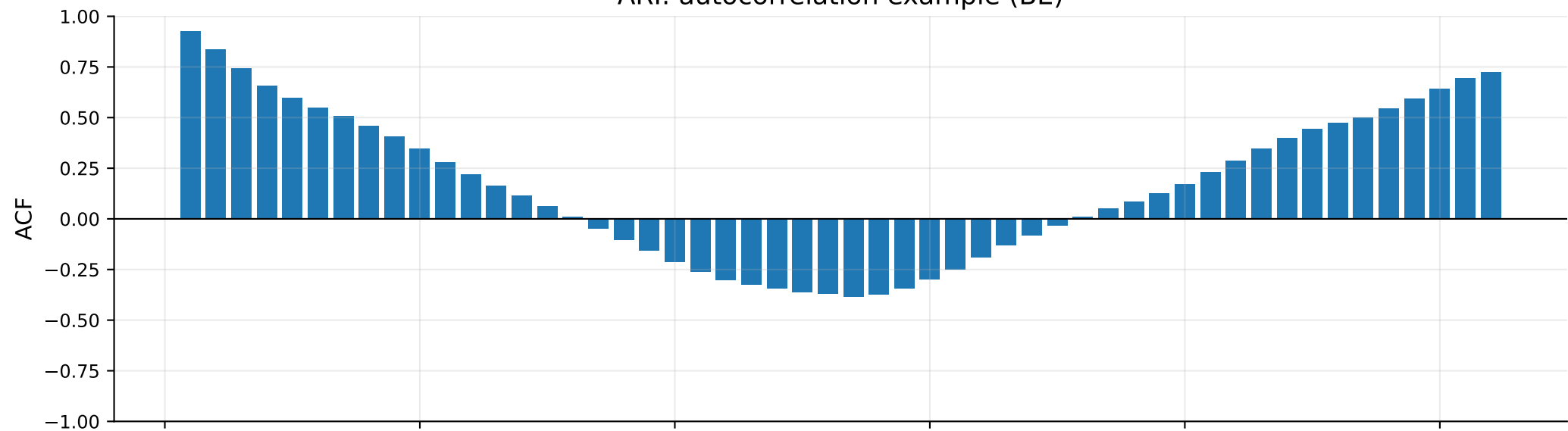
ILI: autocorrelation example (BE)
